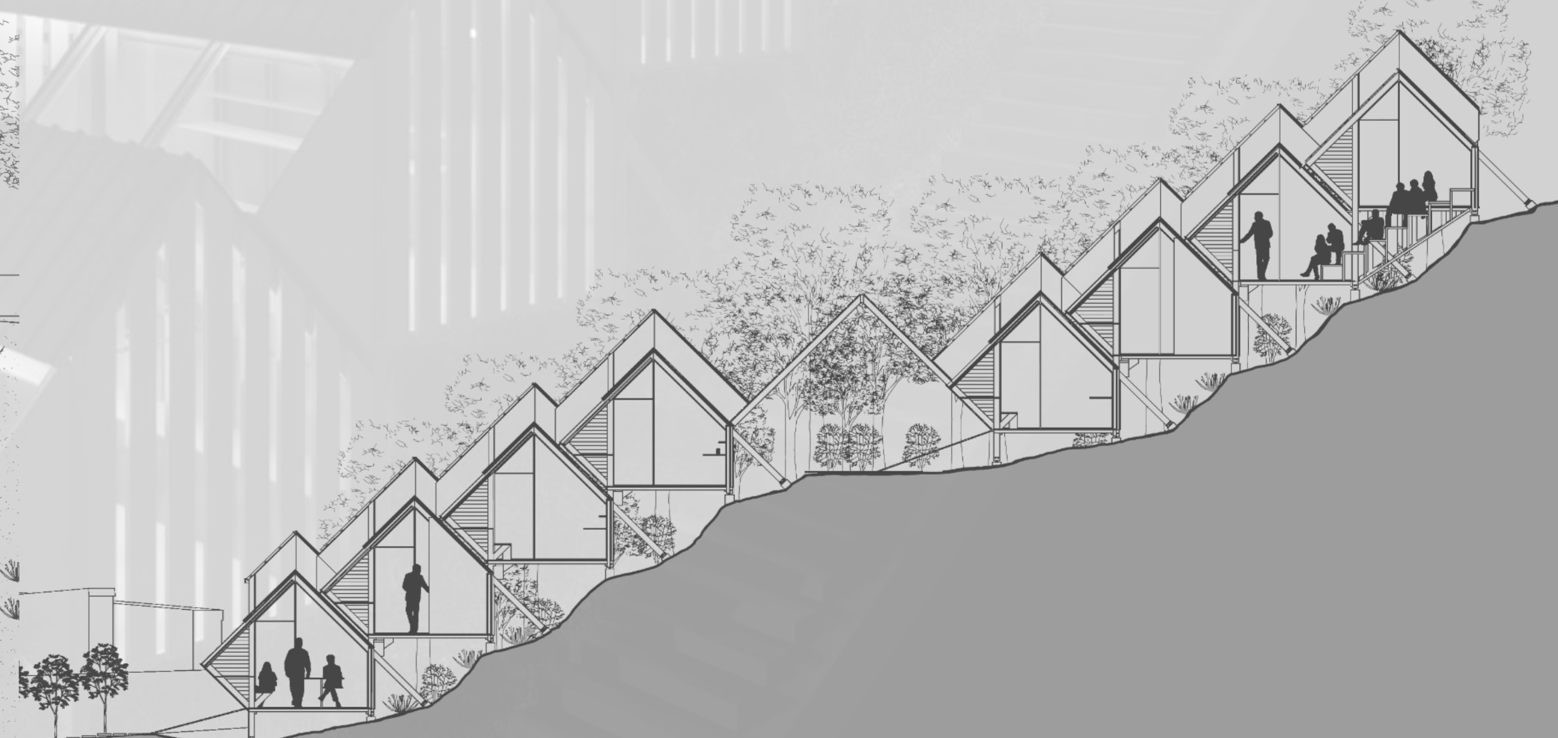
CORTE B-B ESC 1:100
