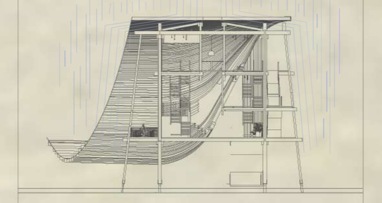
Corte esquemático de caída de Ventilación
