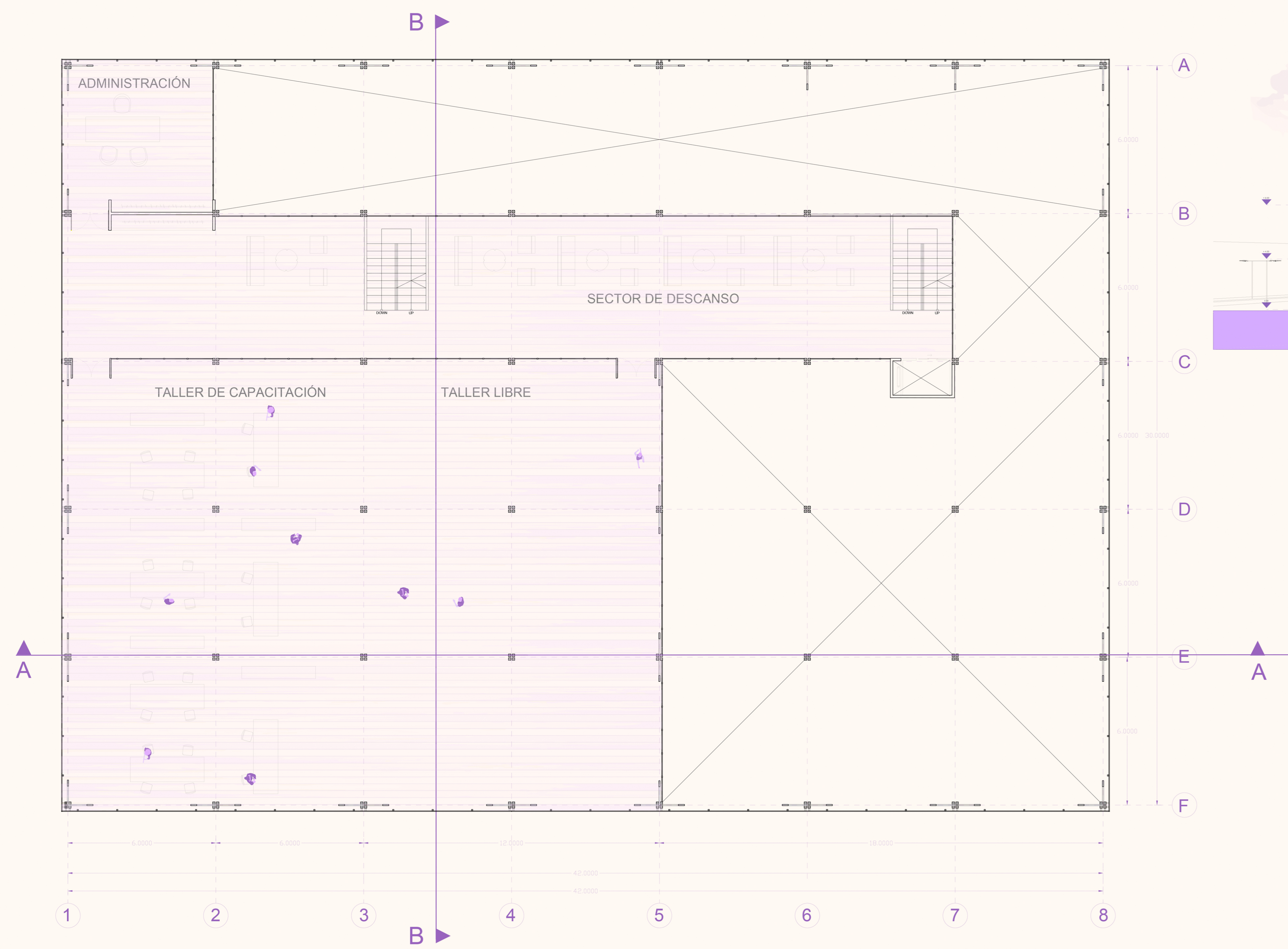
PLANTA SEGUNDO NIVEL ESCALA 1:100
