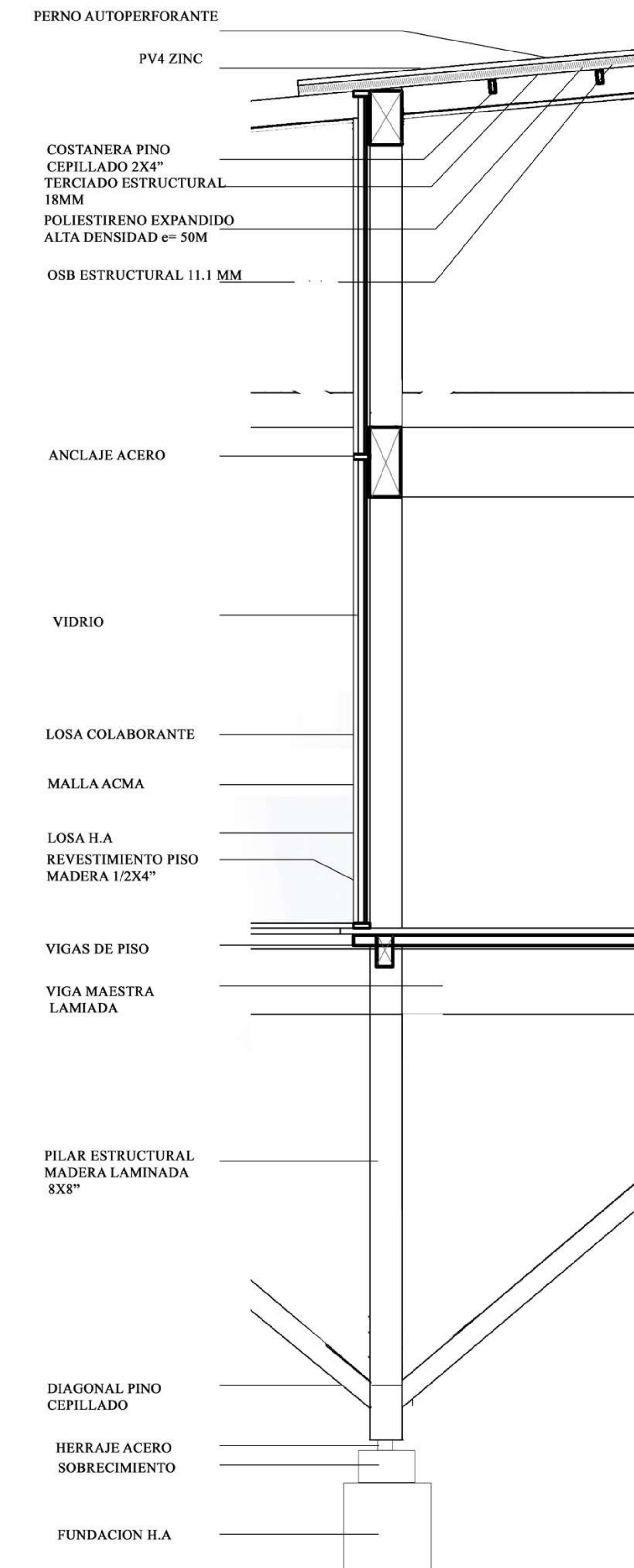
CORTE CONSTRUCTIVO 1:20
