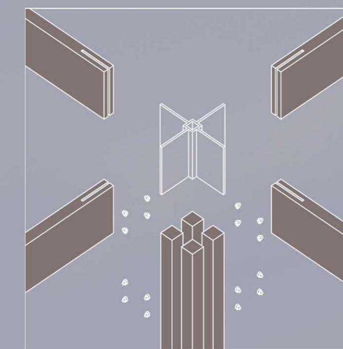
DETALLE EXPLOTADO
