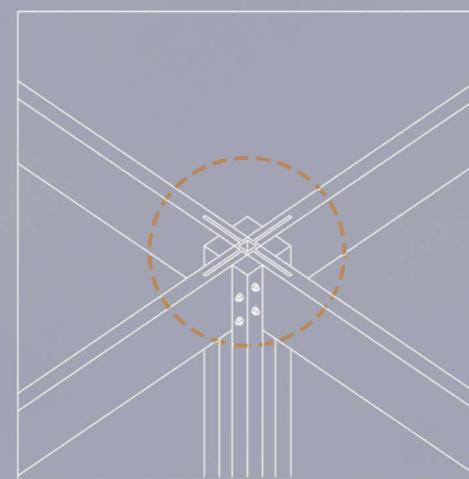
UNIÓN METALICA
