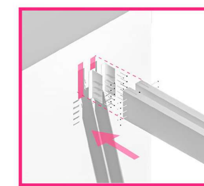
DETALLE VIGA - MURO
