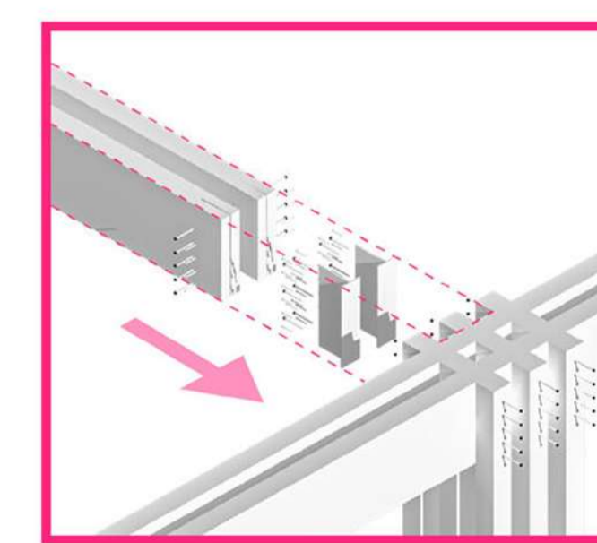
DETALLE VIGA - PILAR
