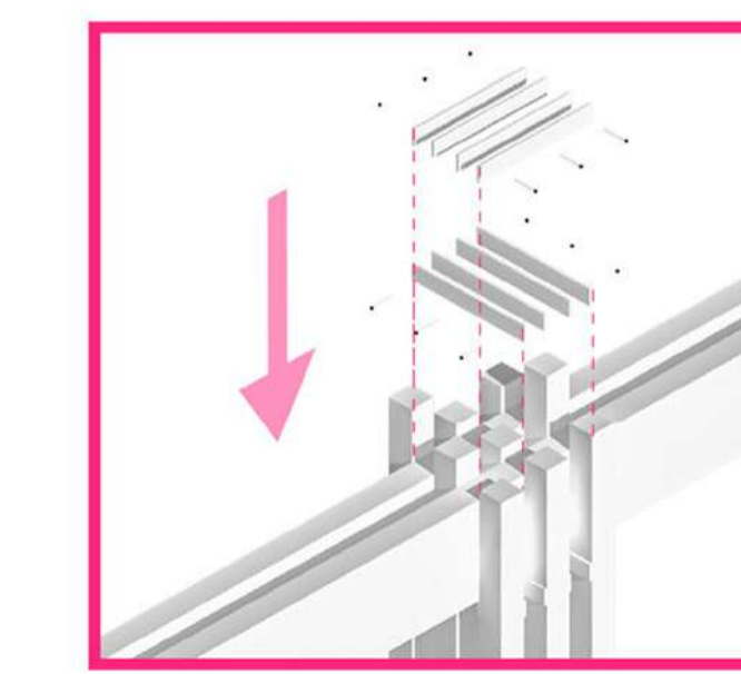
DETALLE PILAR AISLADO
