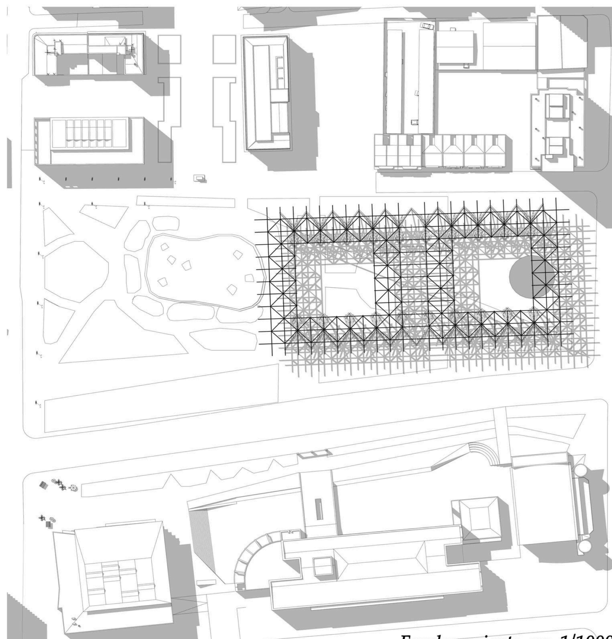
Emplazamiento esc. 1/1000
