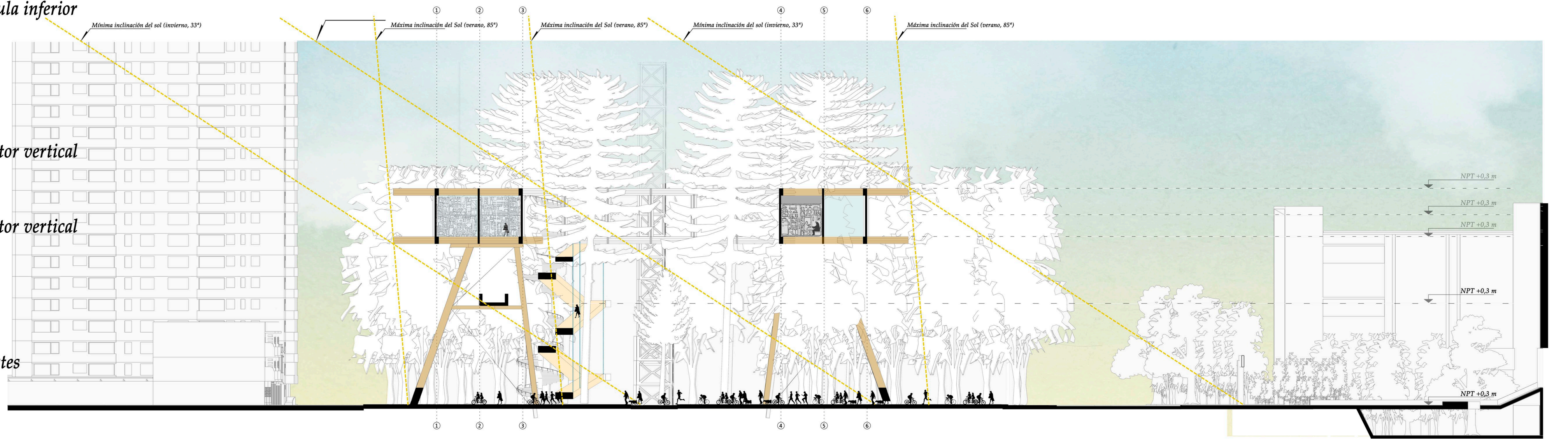
sección B-B' 1:200
