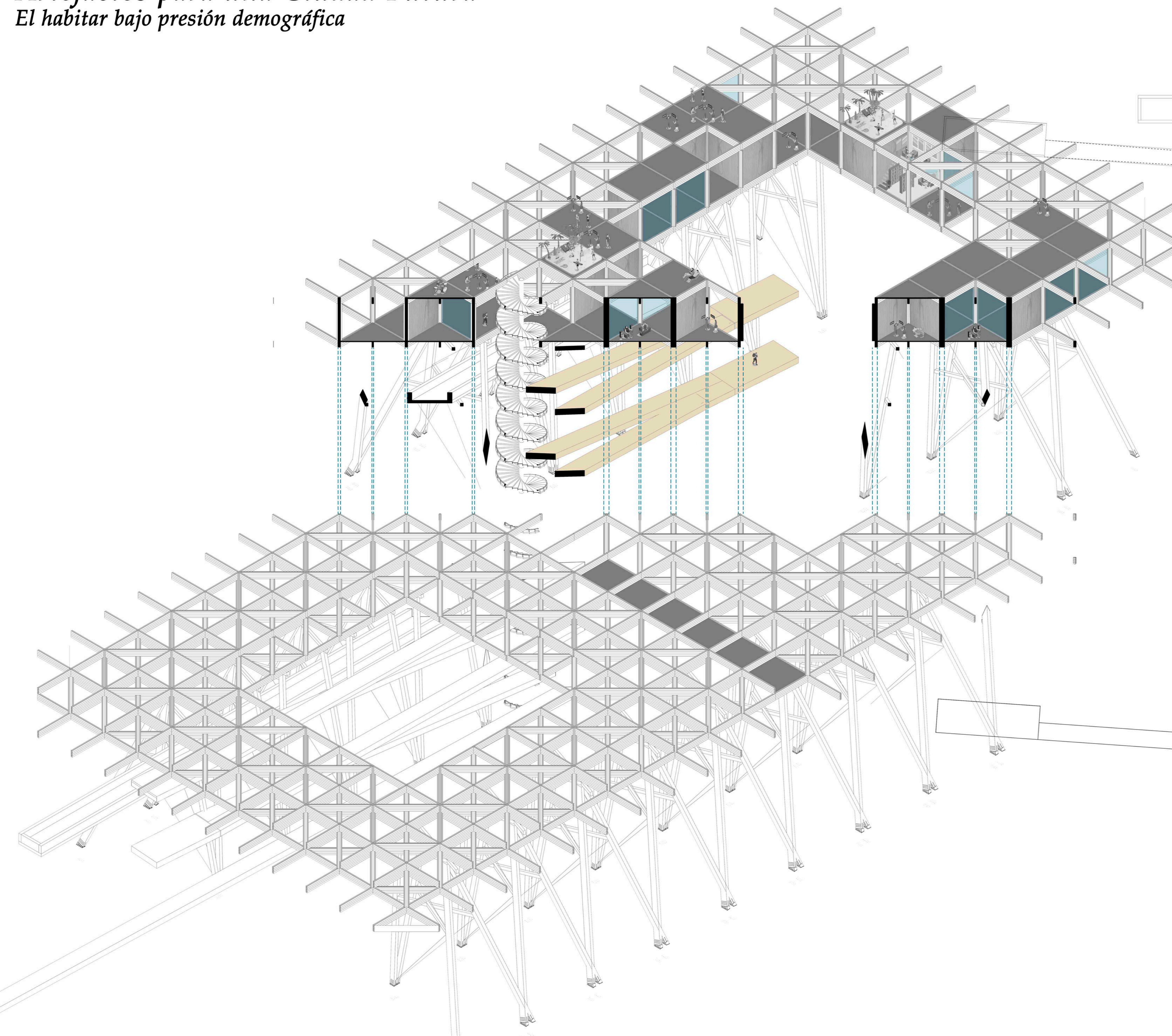
corte isométrico C-C'
