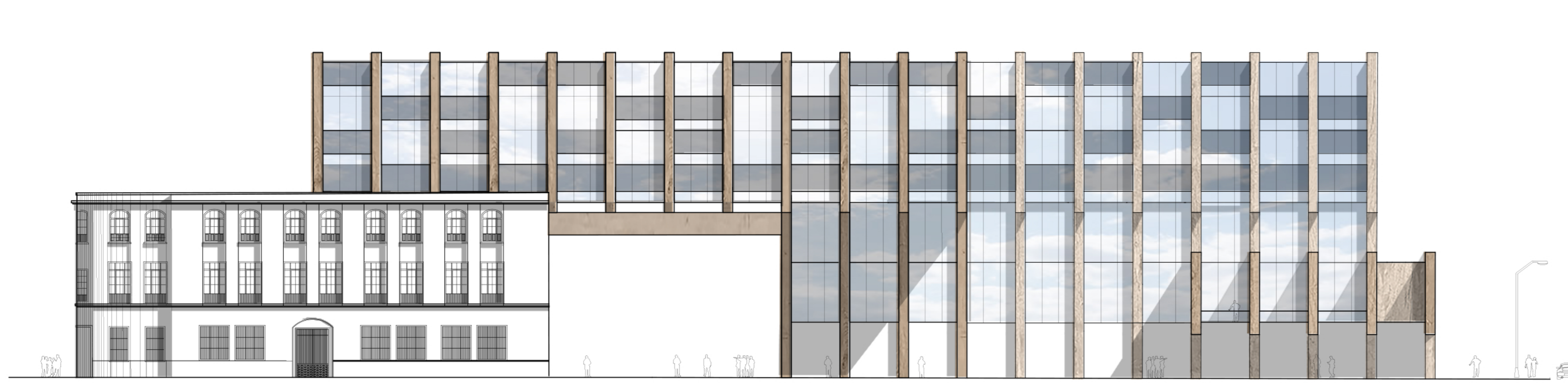
ELEVACION NORTE
