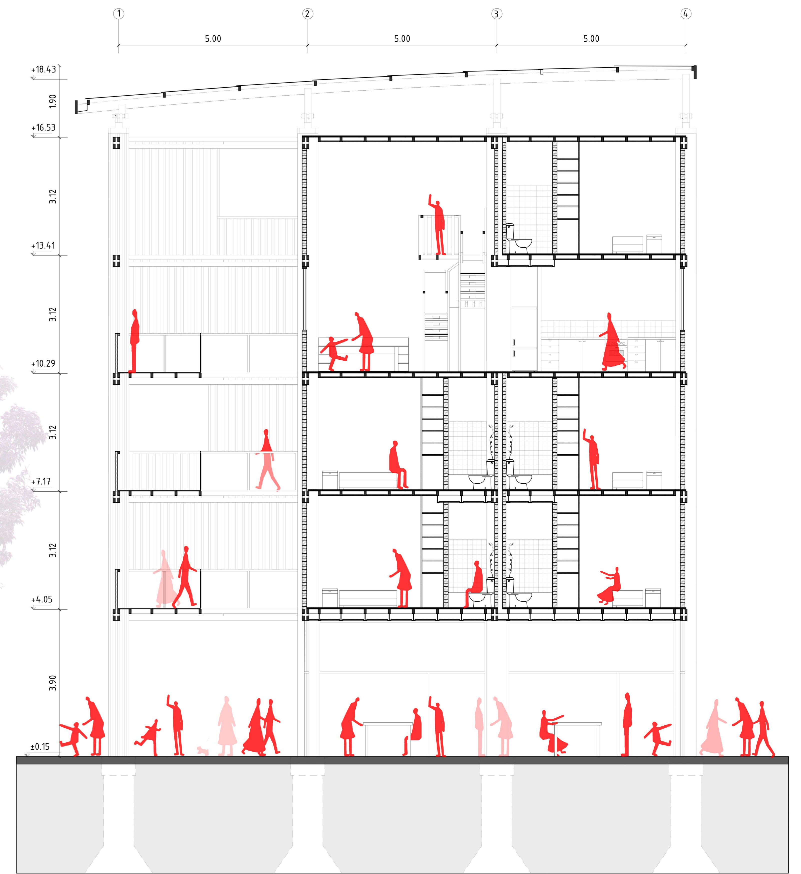
CORTE A-A ESC. 1:50
