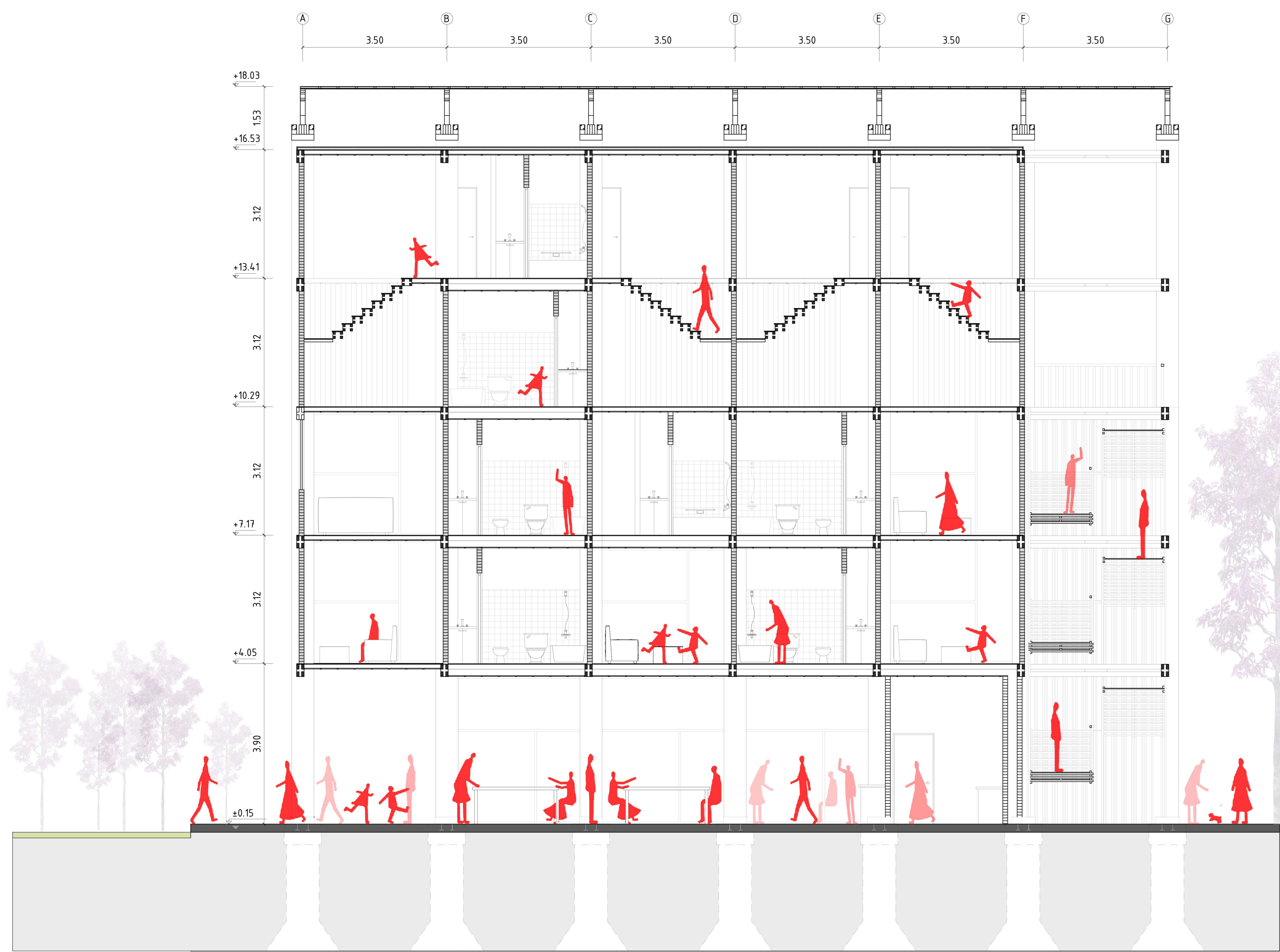
CORTE A-A CONCURSO ARQUITECTURA MADERA21 - CORMA 2018 ARQ-281
