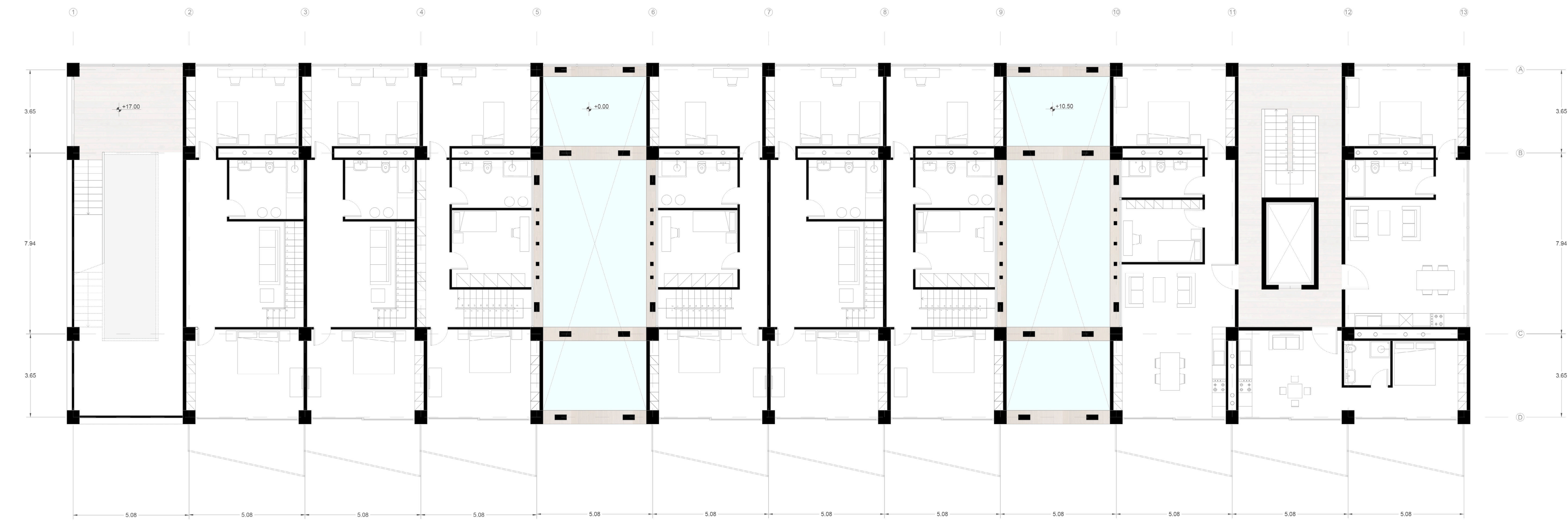
PLANTA CUARTO PISO escala 1:100
