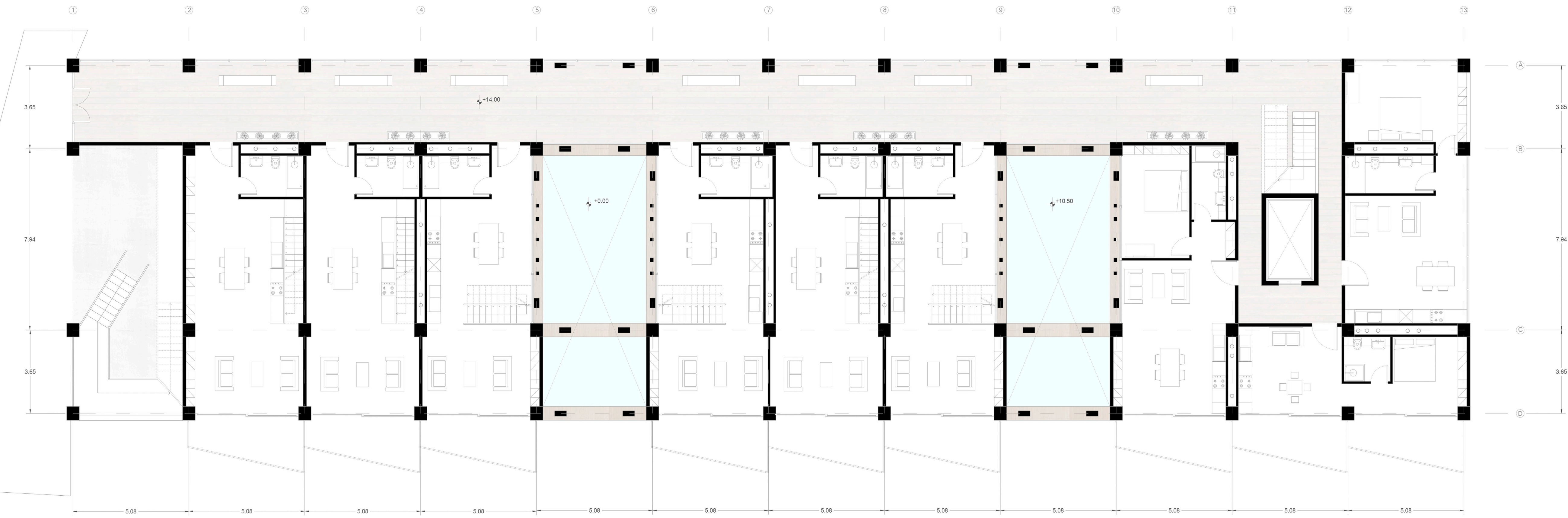
PLANTA TERCER PISO escala 1:100
