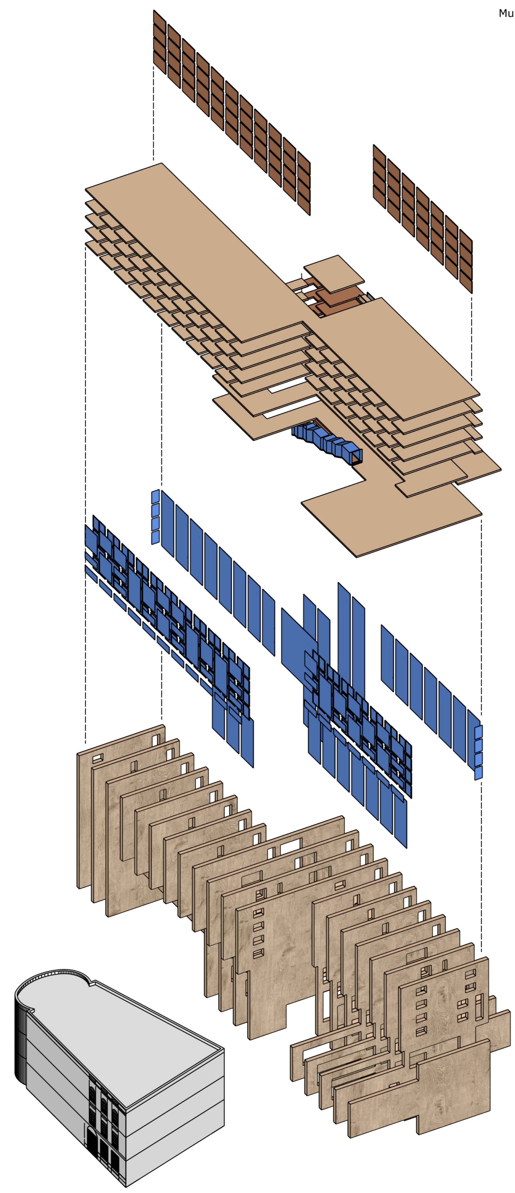
ELEMENTO RIGIDIZADOR (MUROS VIVIENDAS)
