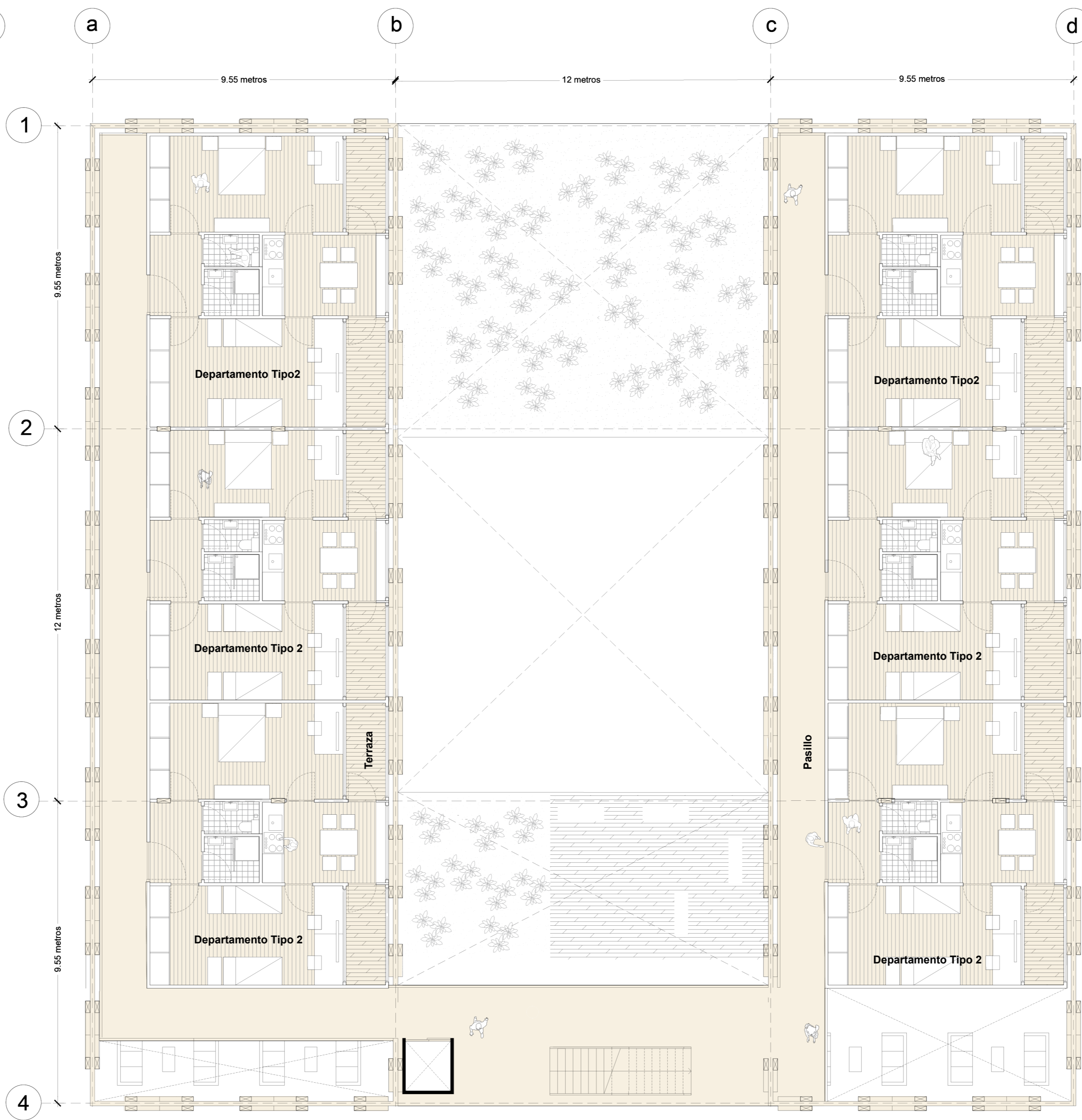
Planta Nivel 3-4 esc 1:100
