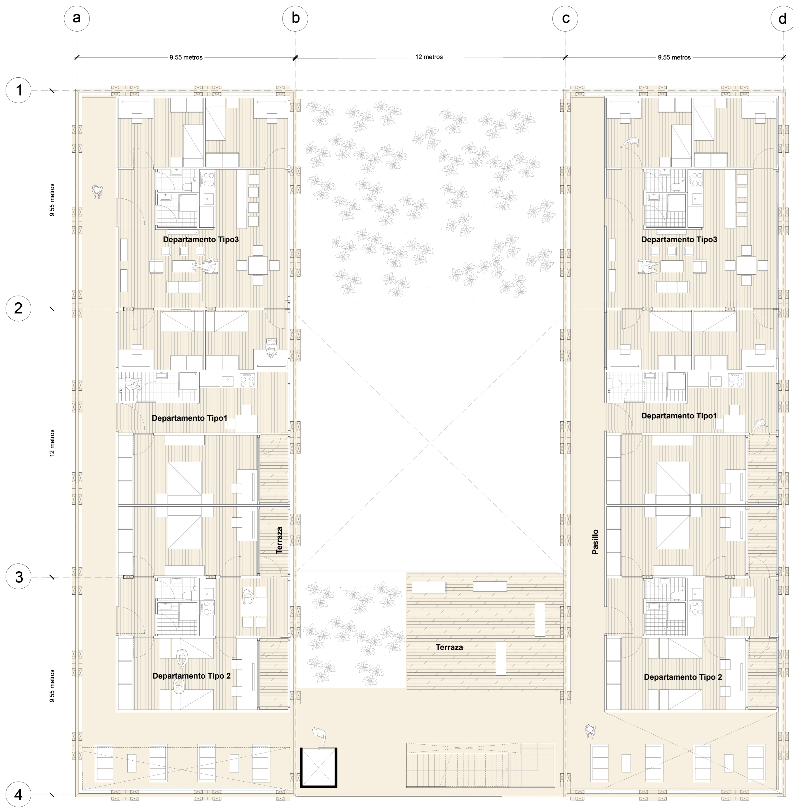
Planta Nivel 2 esc 1:100
