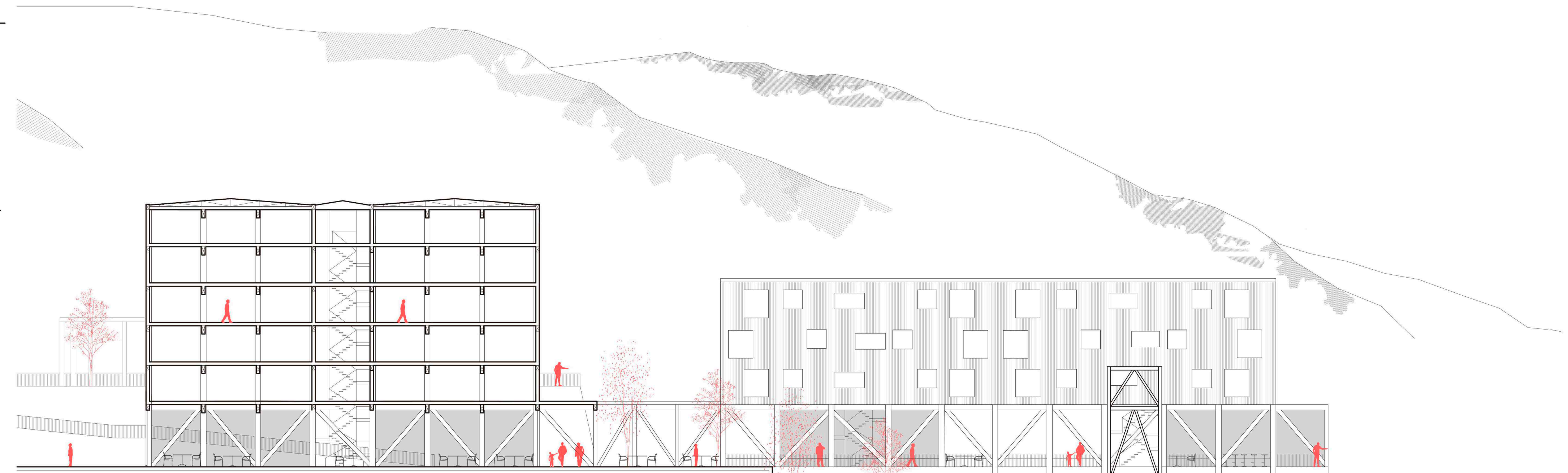
CORTE TRANSVERSAL A-A 1:200
