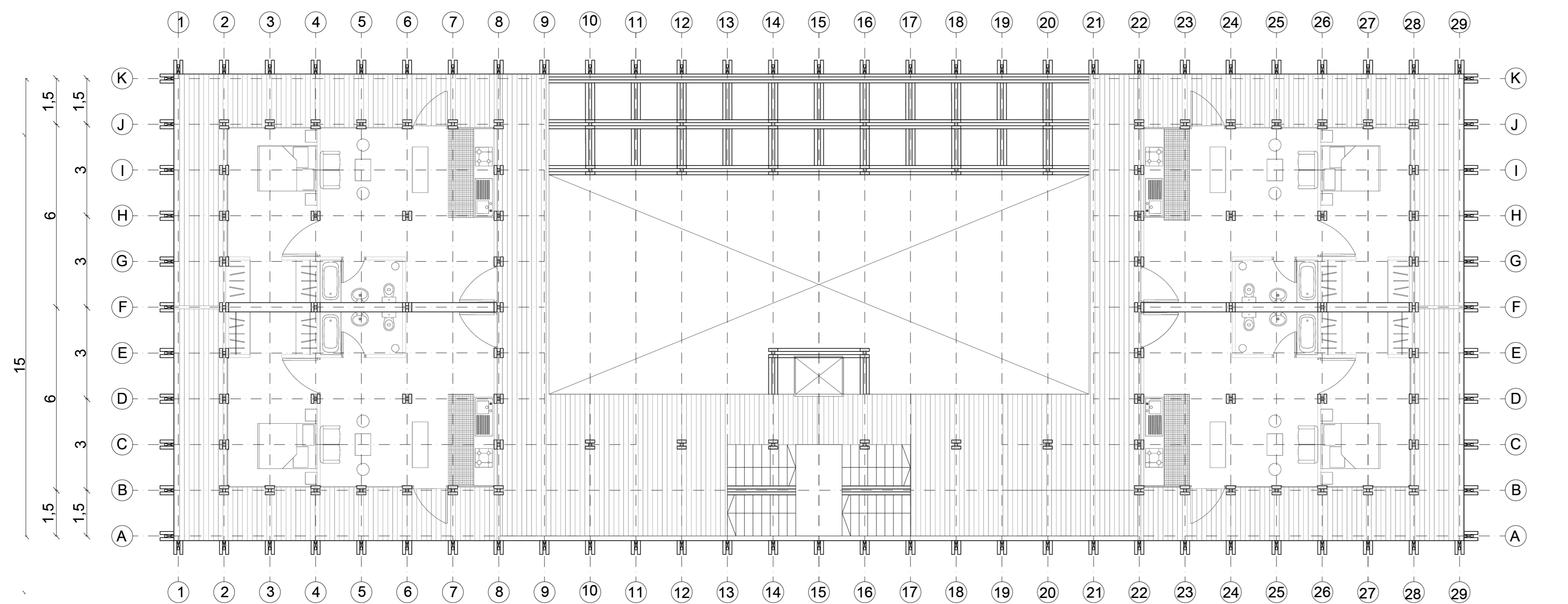
PLANTA NVL.3 ESC. 1:100
