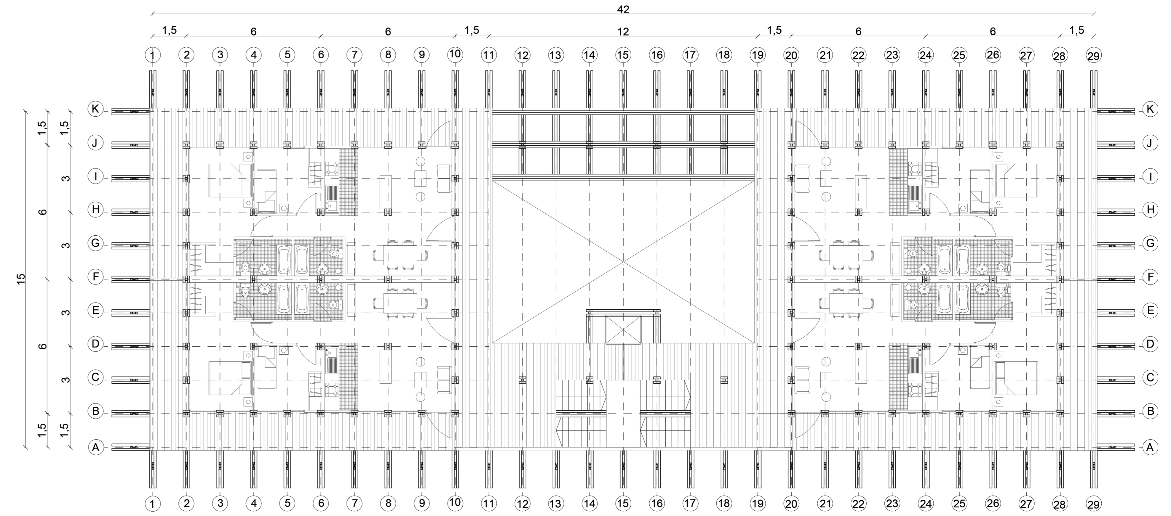
PLANTA NVL.4 ESC. 1:100
