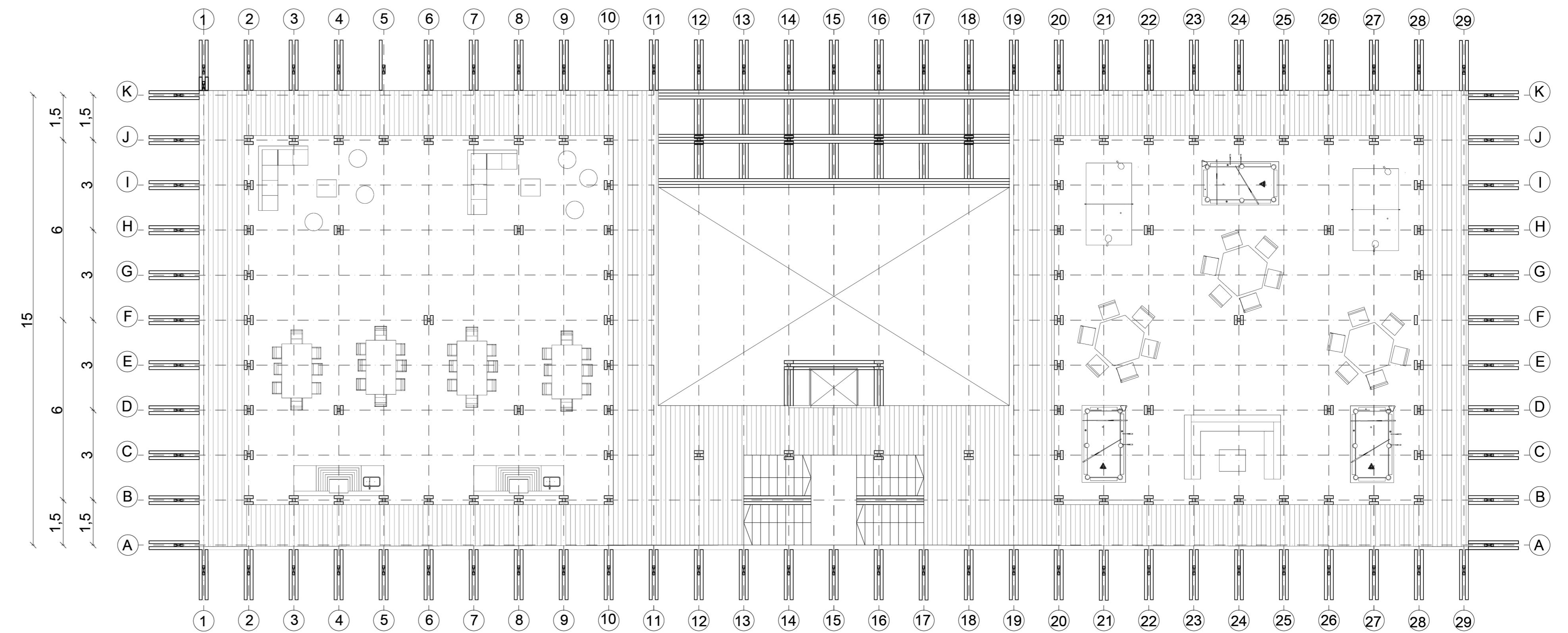
PLANTA NVL.5 ESC. 1:100
