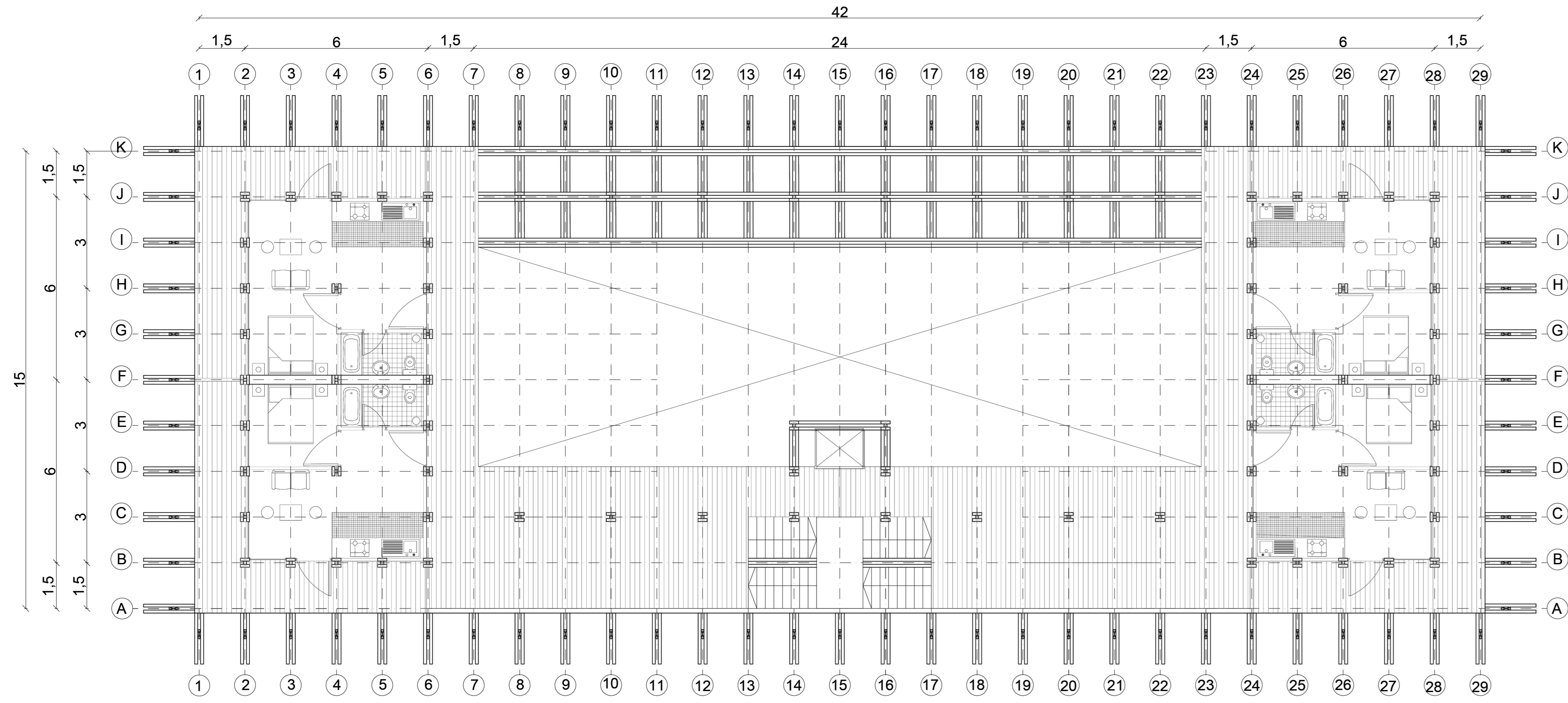
PLANTA NVL.2 ESC. 1:100
