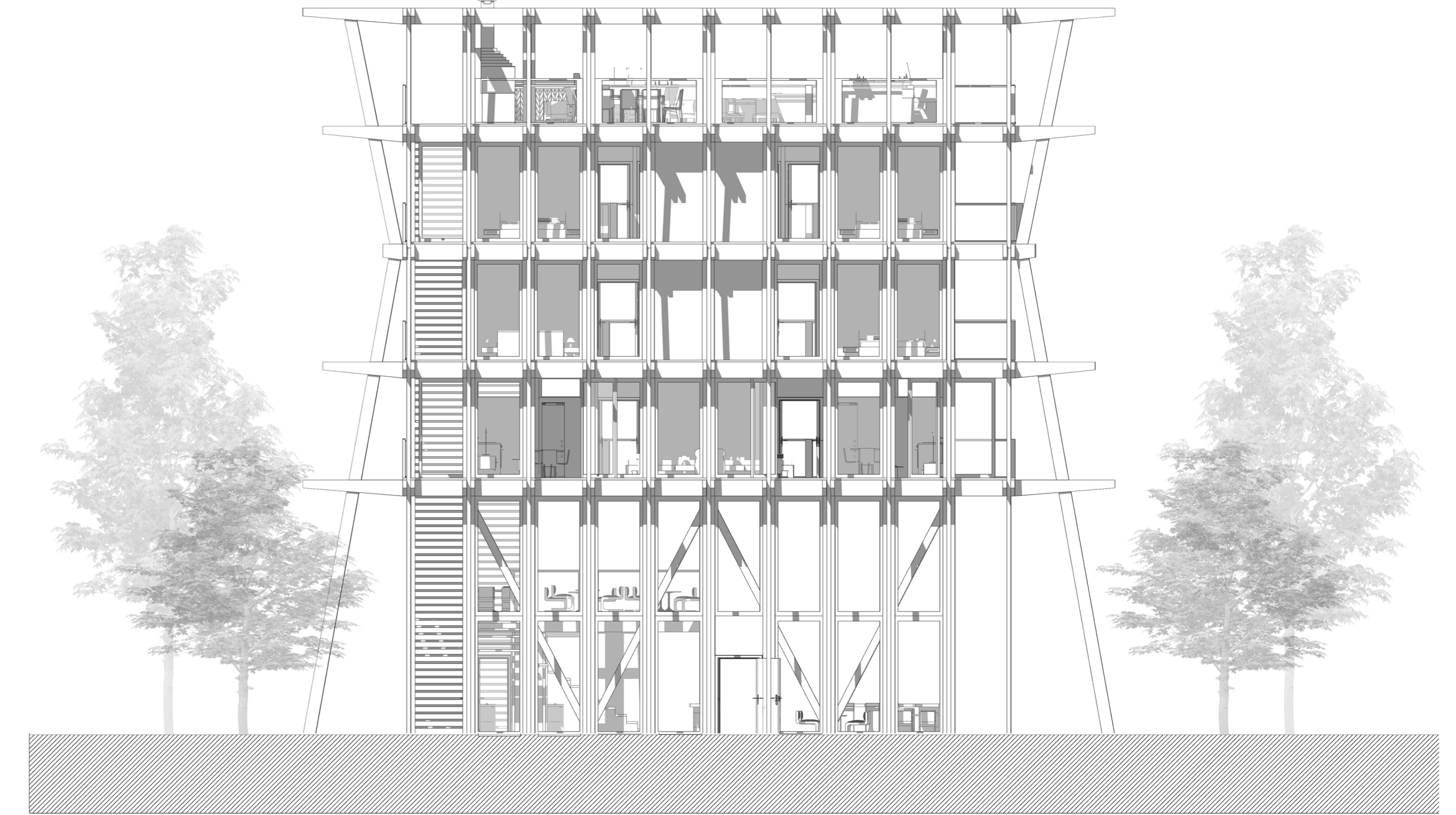
ELEVACIÓN SUR ESC. 1:100
