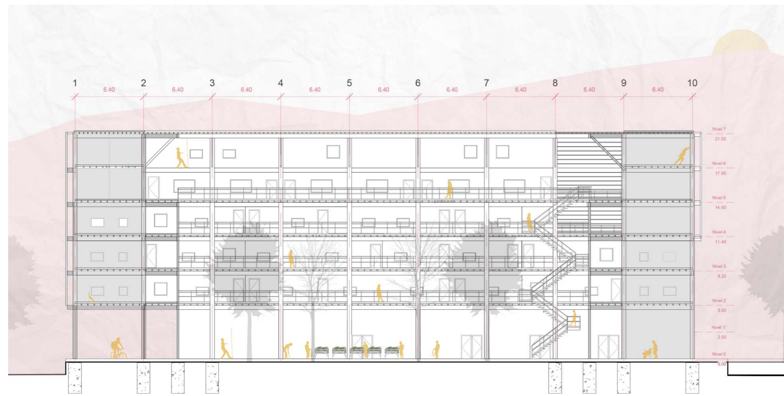
CORTE AA' - ESCALA 1:200
