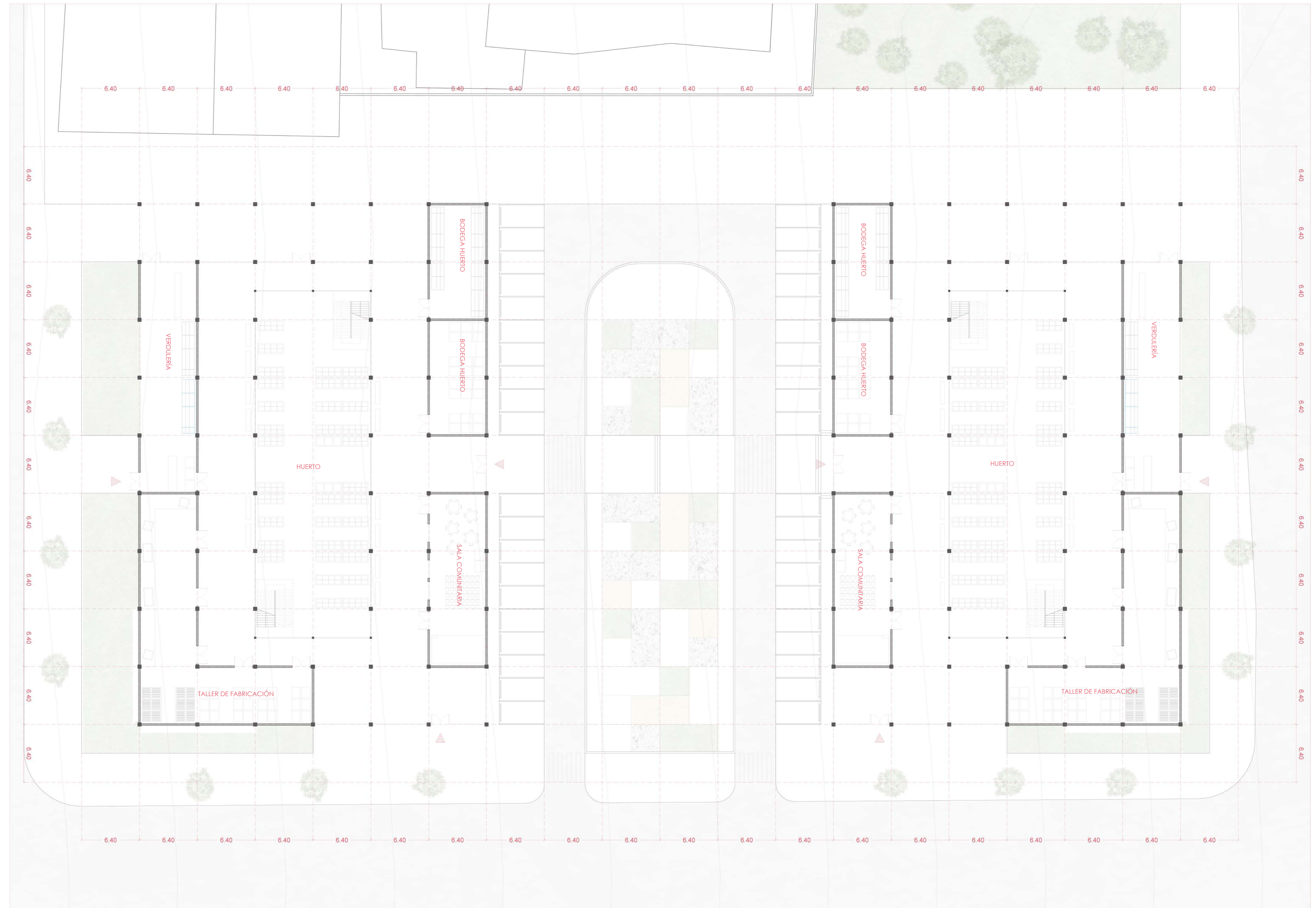
PLANTA NIVEL 1 - ESCALA 1:200
