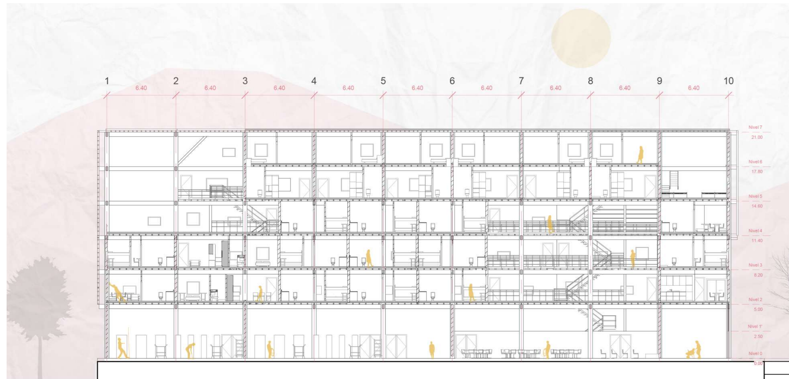
CORTE CC' - ESCALA 1:200
