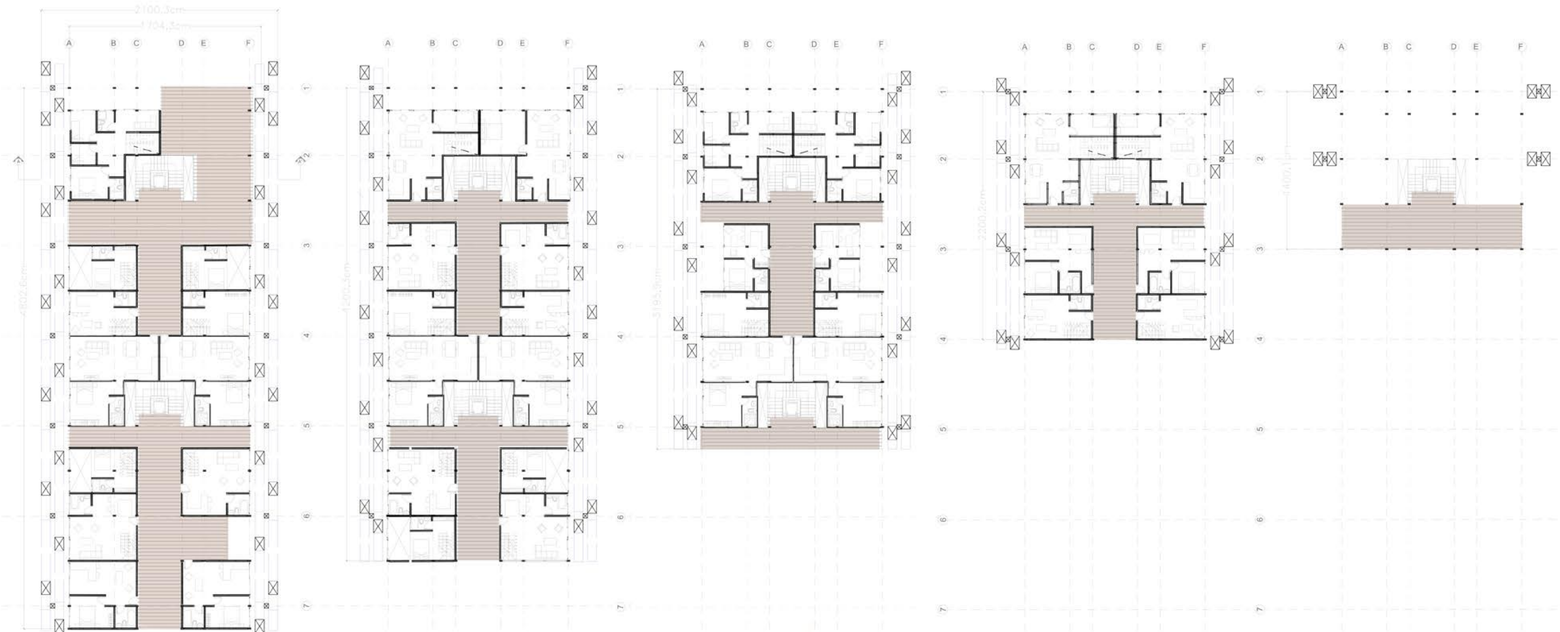
PLANTA 5TO PISO / BLOQUE 2 esc 1:200
