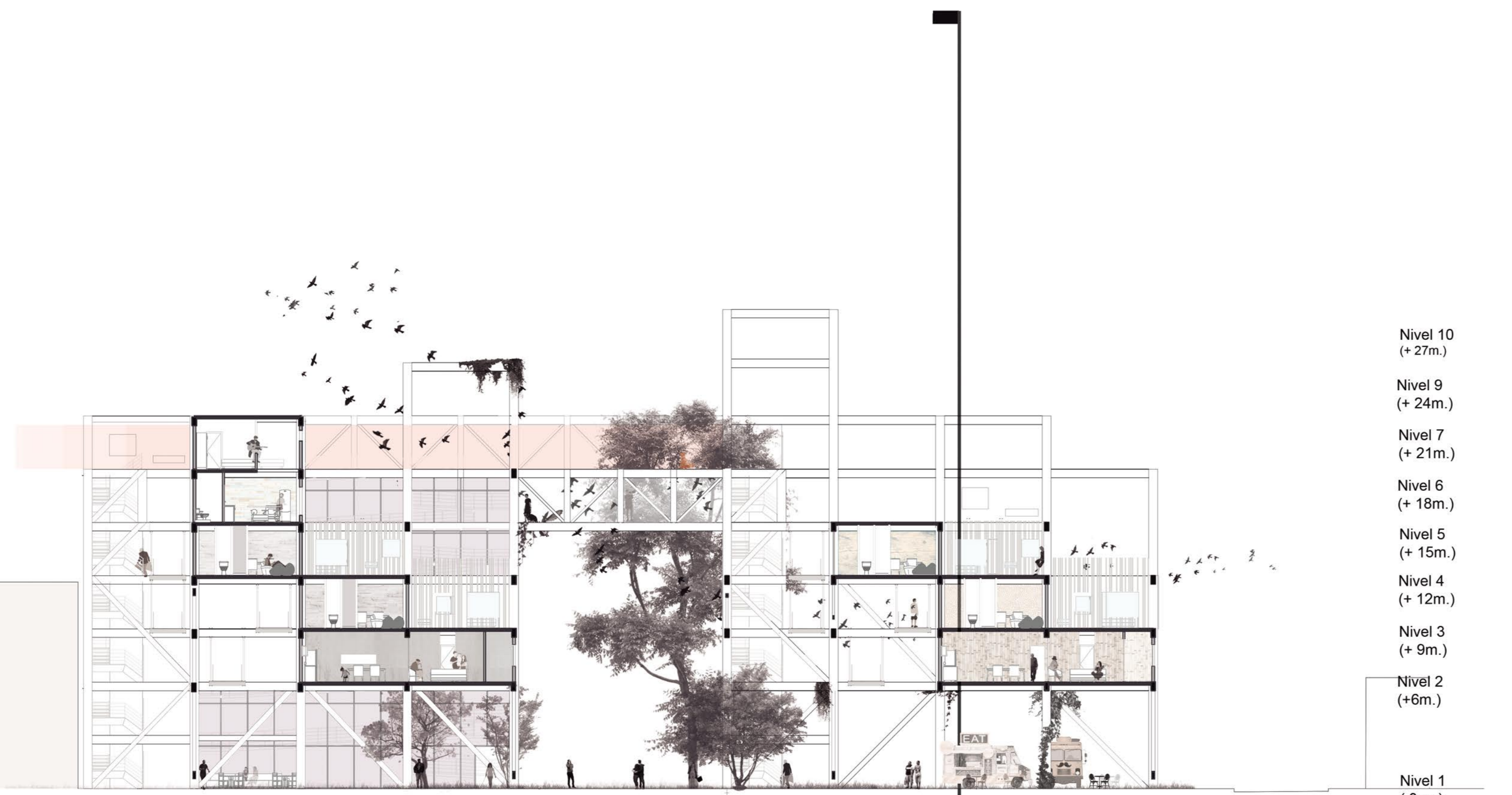
CORTE A'-A Esc 1:200
