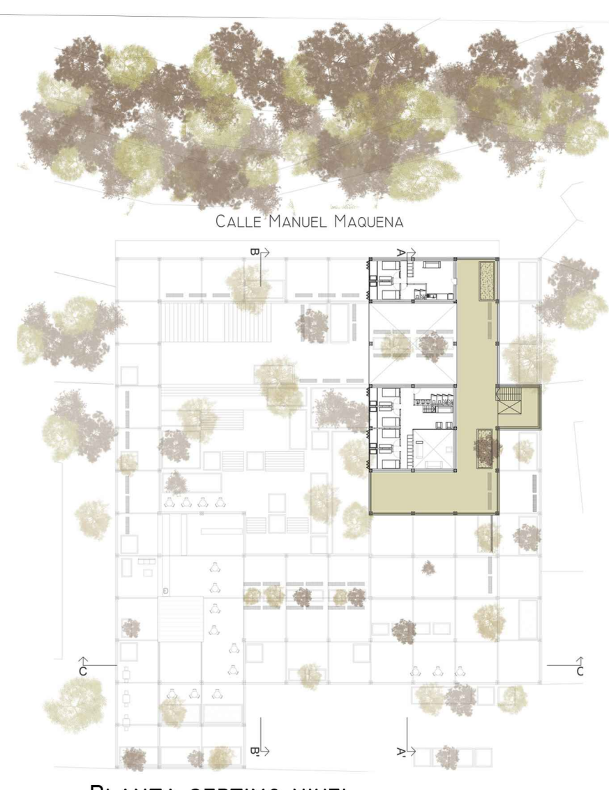
PLANTA SEPTIMO NIVEL
