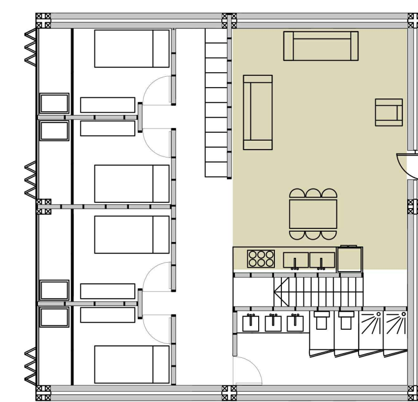
TIPOLOGIA DE VIVIENDA - DUPLEX ESCALA 1:100
