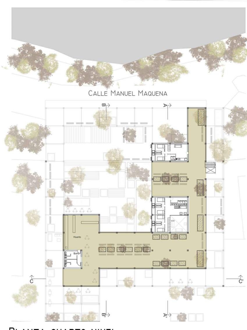
PLANTA CUARTO NIVEL
