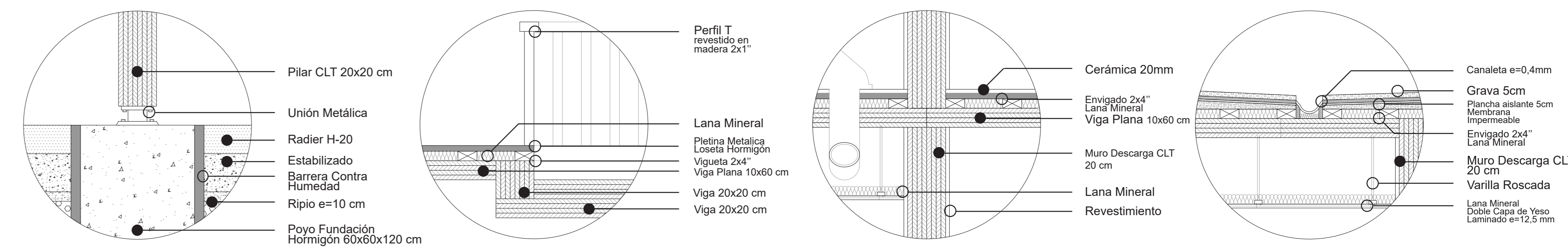
Detalle 1 Anclaje Fundación Detalle 2 Veranda Detalle 3 Muro Descarga Detalle Cubierta Escala 1:15
