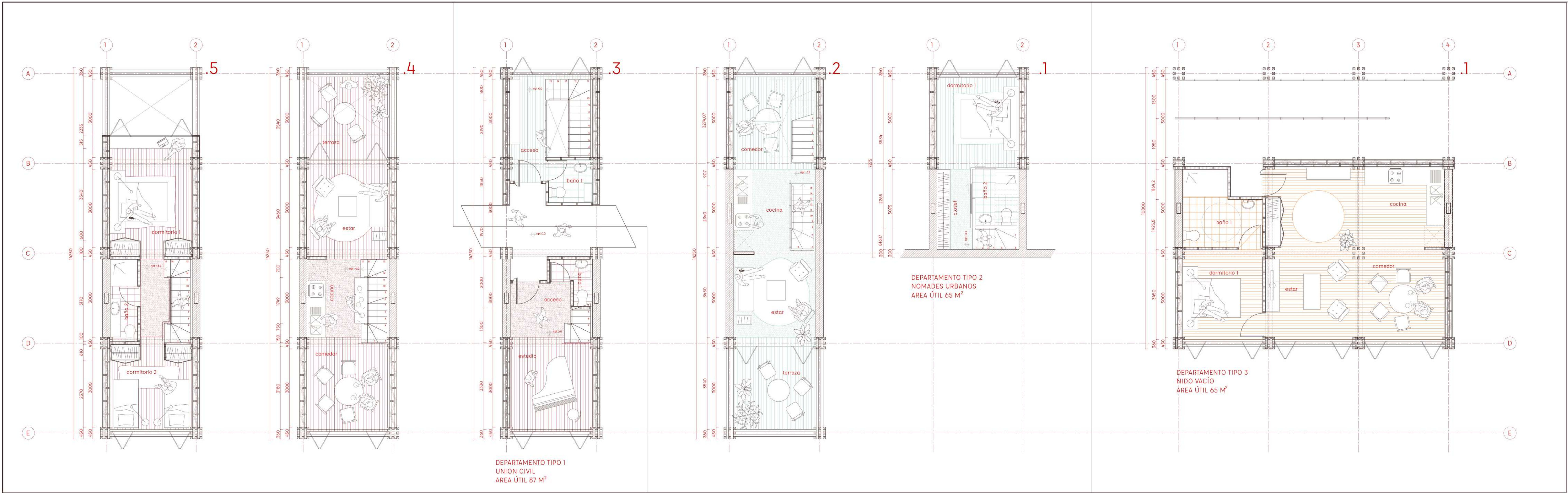
PLANTAS DEPARTAMENTOS TIPO ESCALA 1:75
