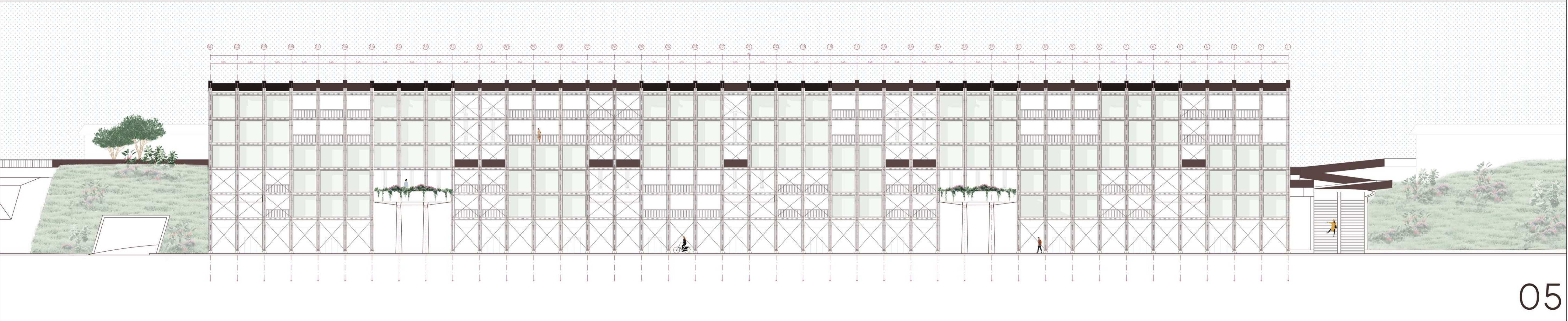
ELEVACION NORTE / NUEVA COSTANERA ELQUI ESCALA 1:250
