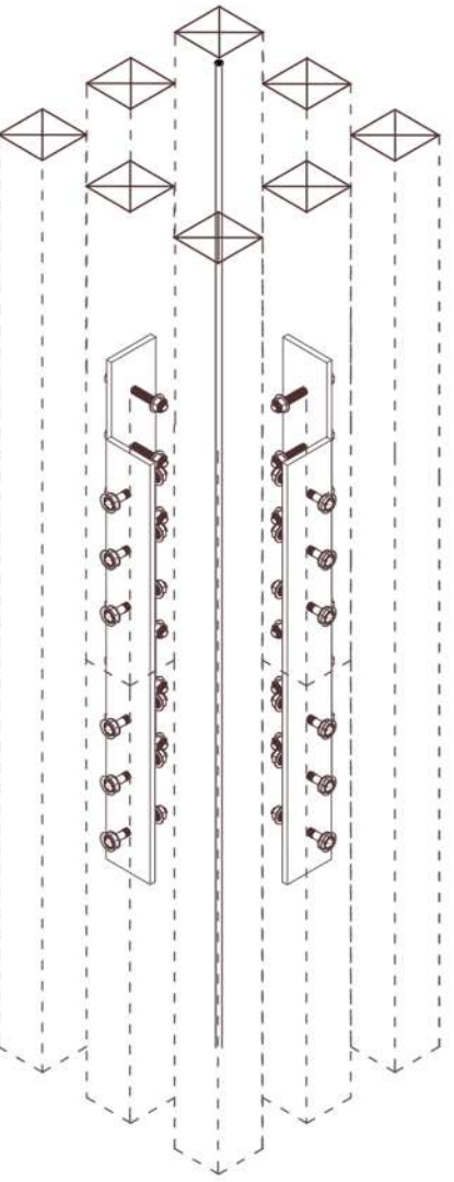
DETALLE 1 UNION VERTICAL PILAR COMPUESTO
