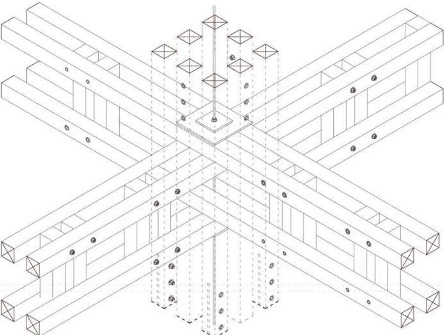
DETALLE 2 UNION HORIZONTAL VIGAS / TENSOR SIMPSON
