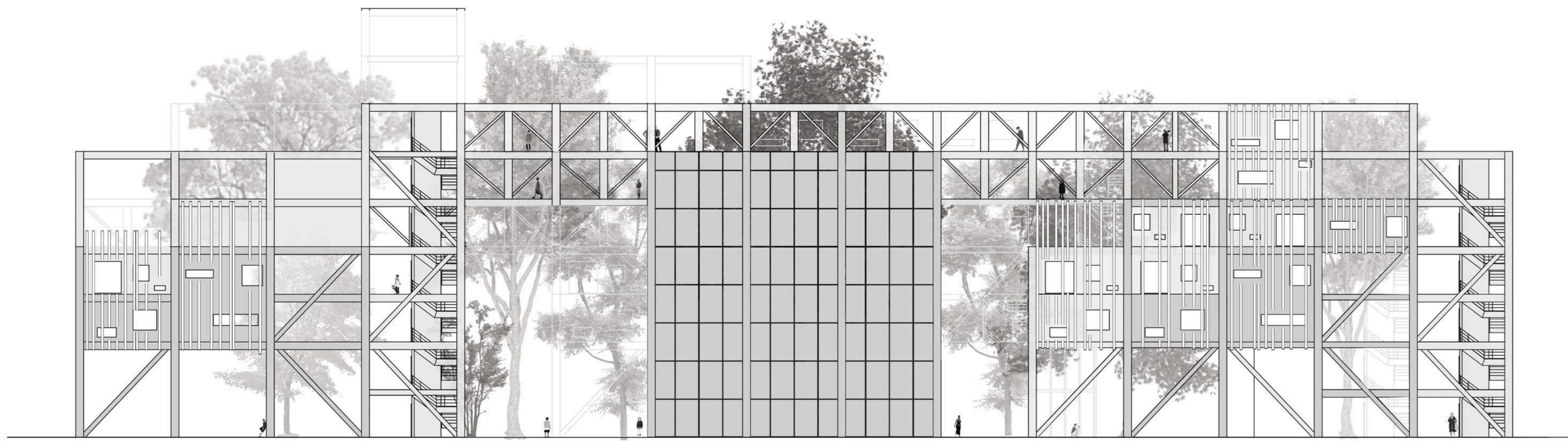
ELEVACION SAN FRANCISCO ESC 1/200
