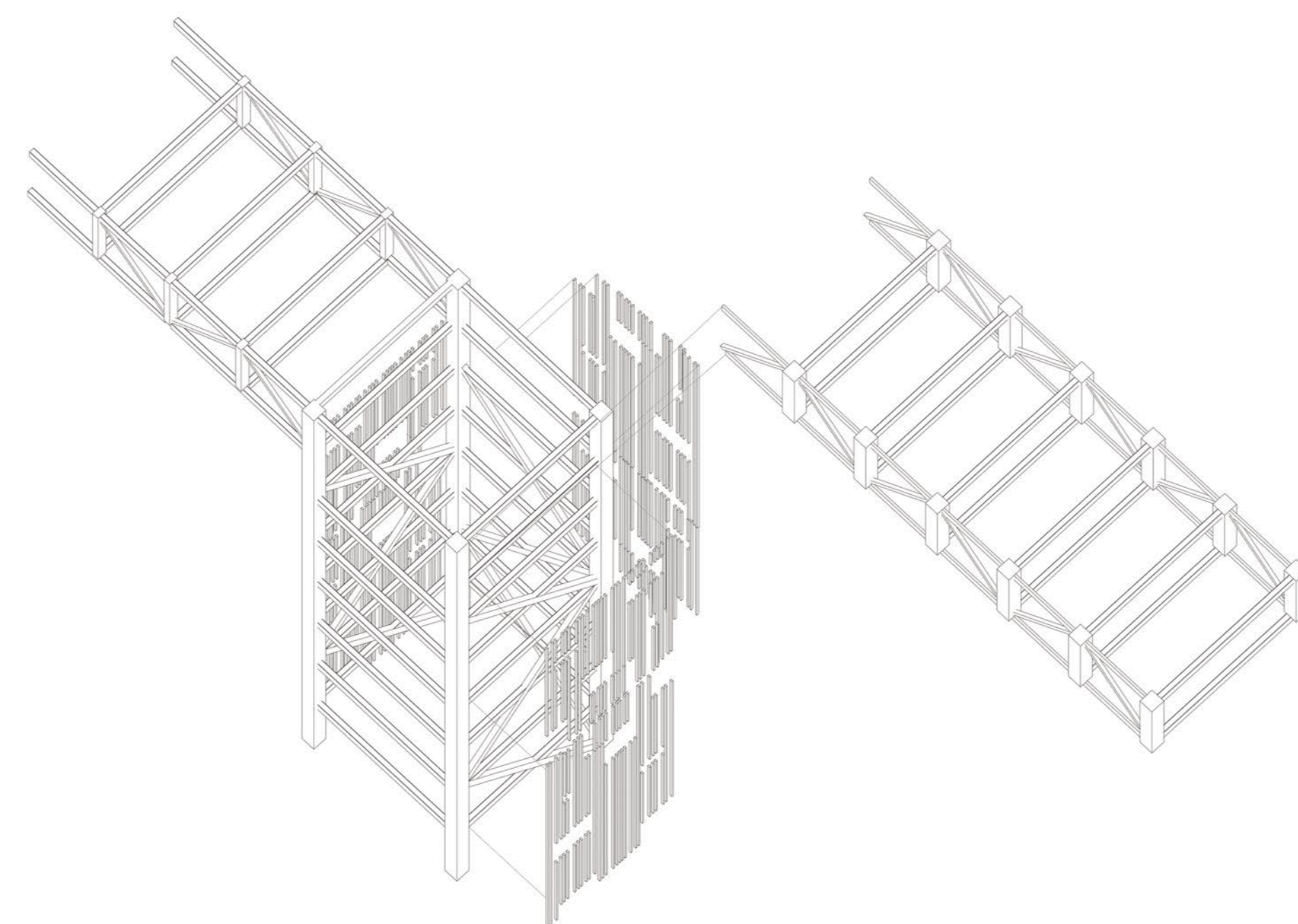
Nucleo vertical explotado
