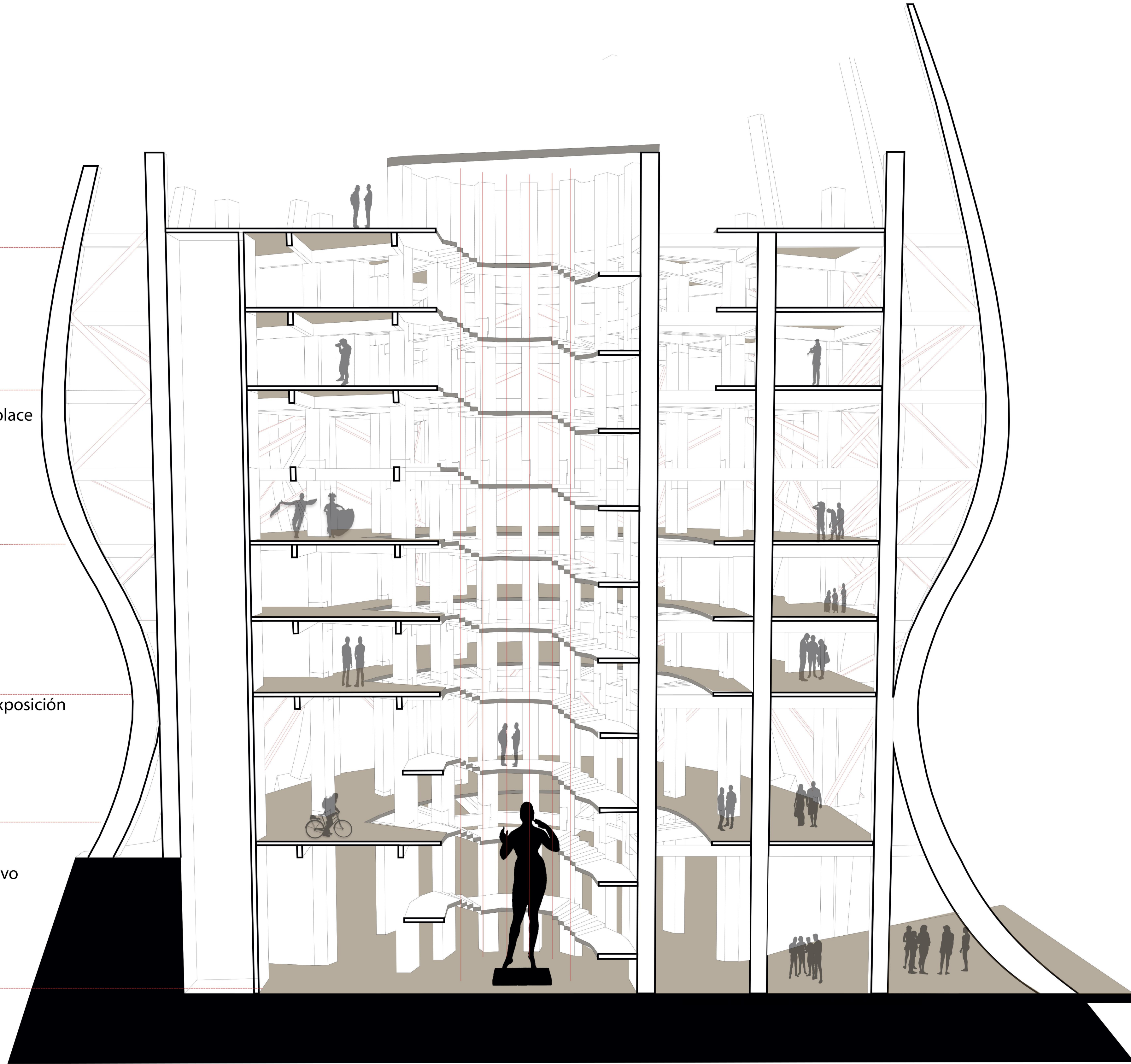
CORTE A-A'
