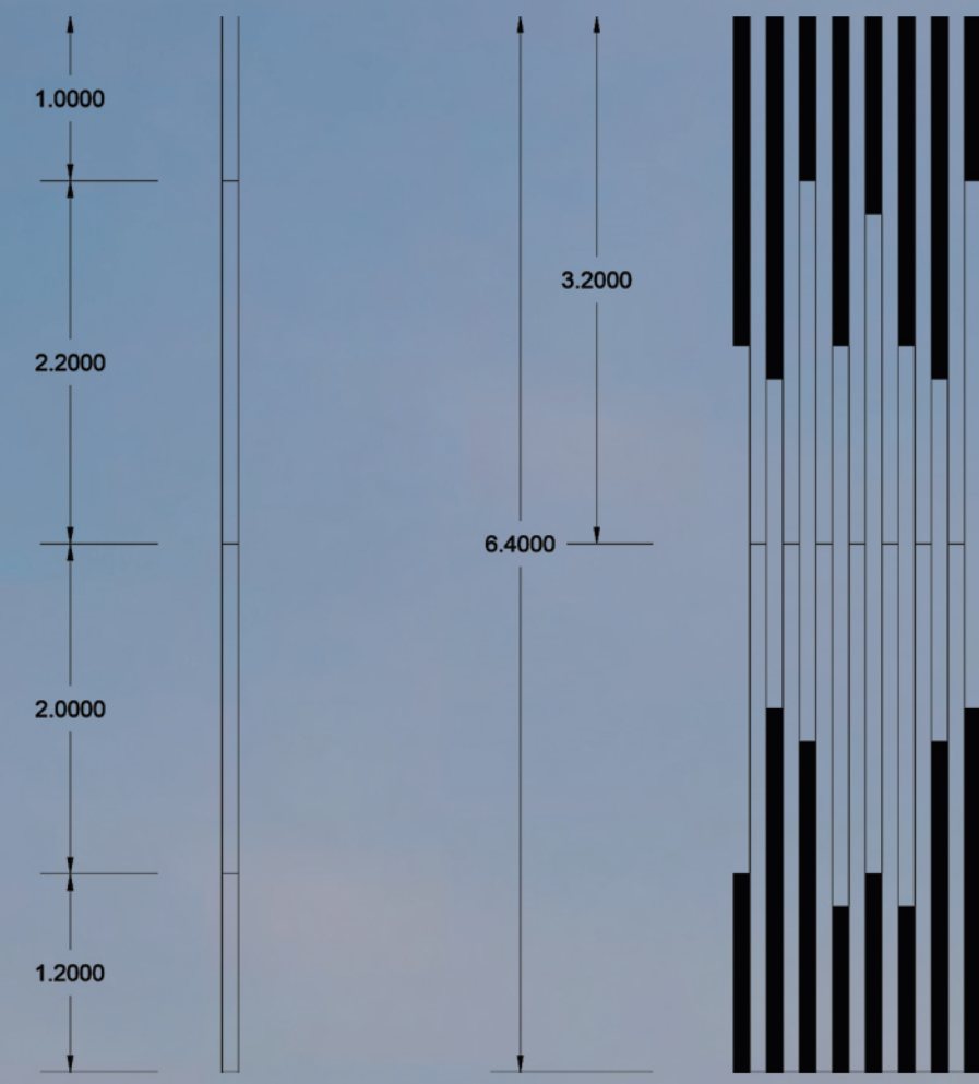
Esquema celosía | ESC 125
