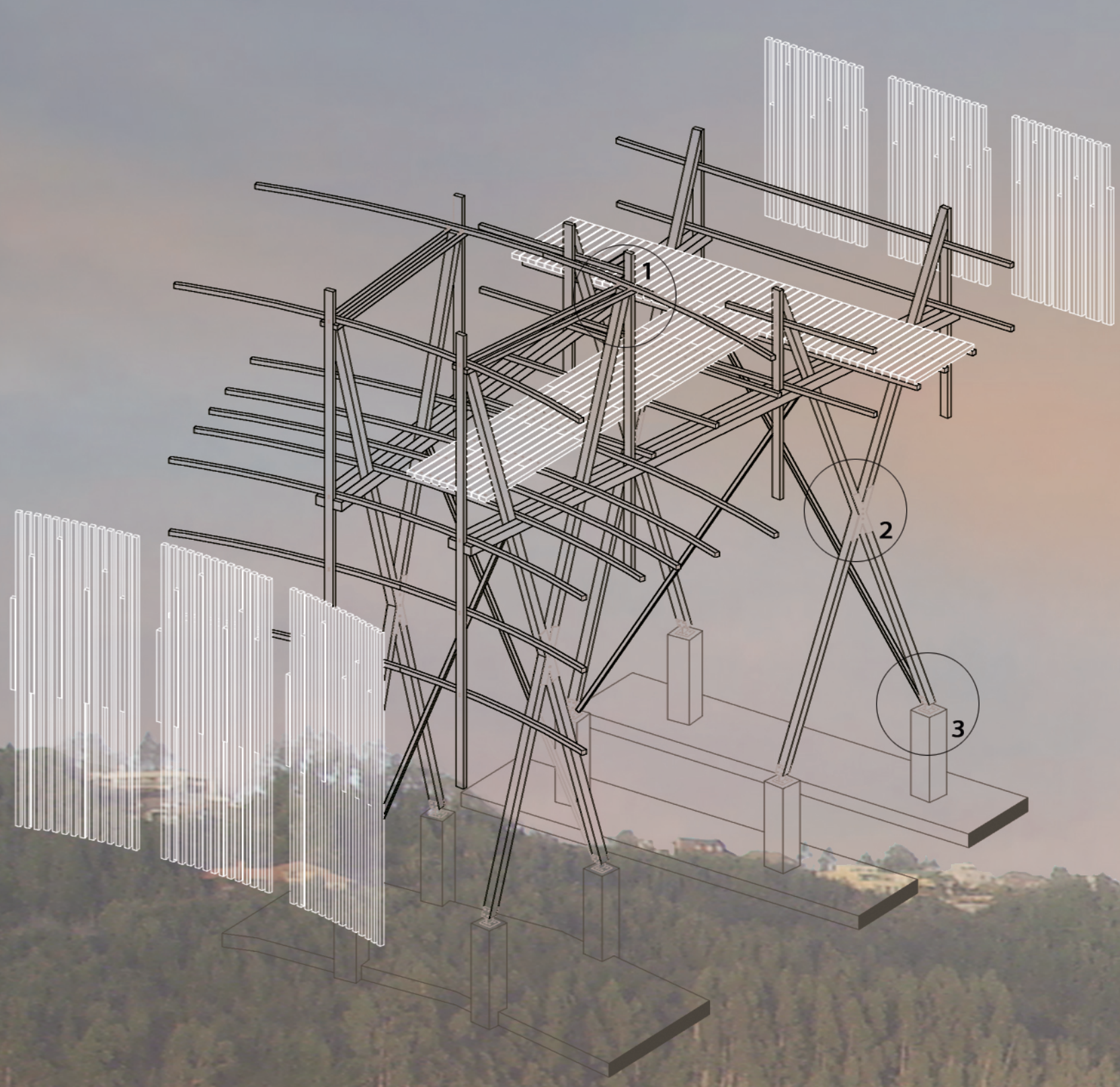
Isométrica sección de unión entre puente y foyer 360
