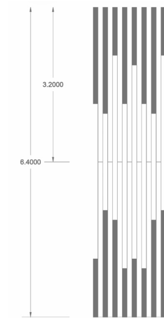
Imagen n°5 Esquema celosía
