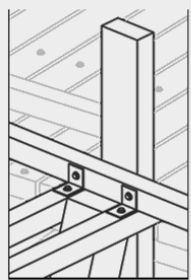
1.-Conexión entre dos piezas con pernos de 1 1/2"
