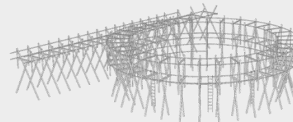
Pilares compuestos en "X"
