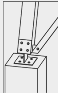
3.-Unión entre fundación y pilar con pernos de 3/8"
