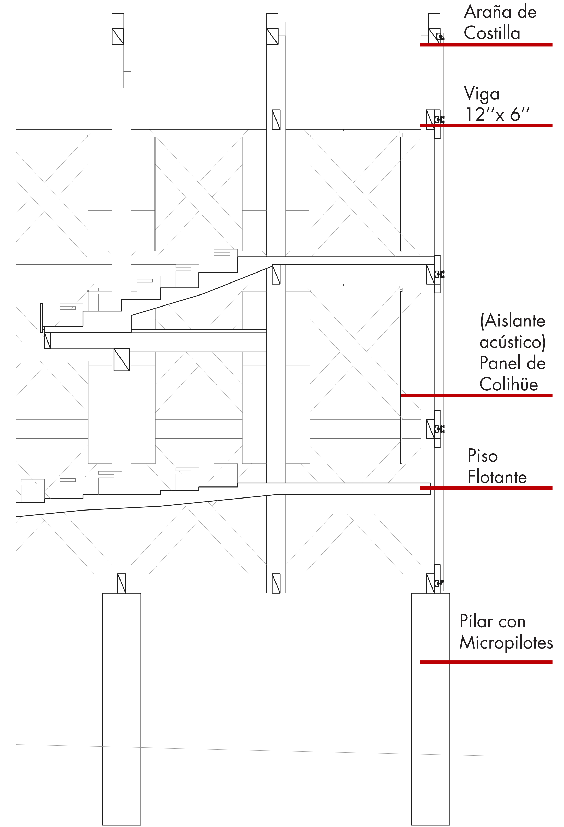
Escantillón 1.25
