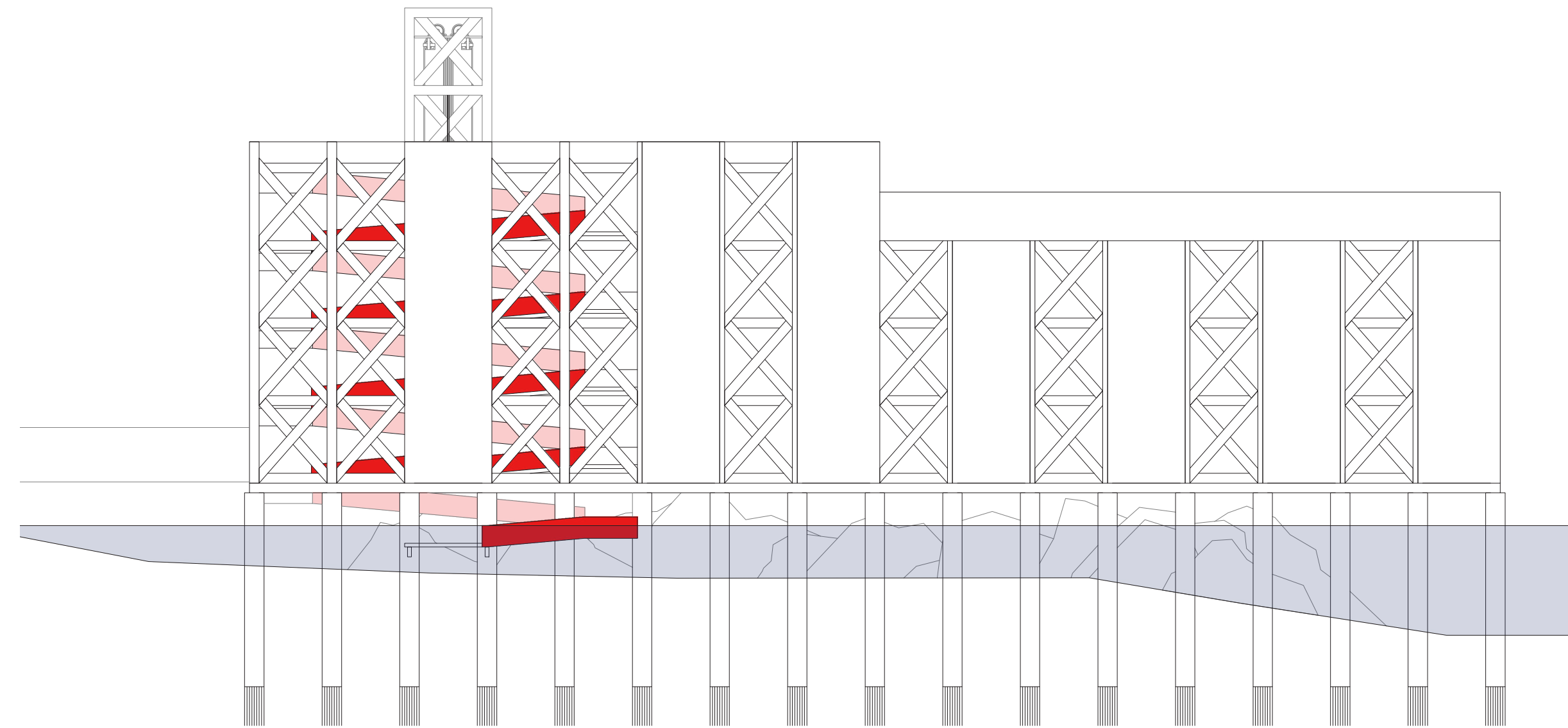
Elevación 1.250
