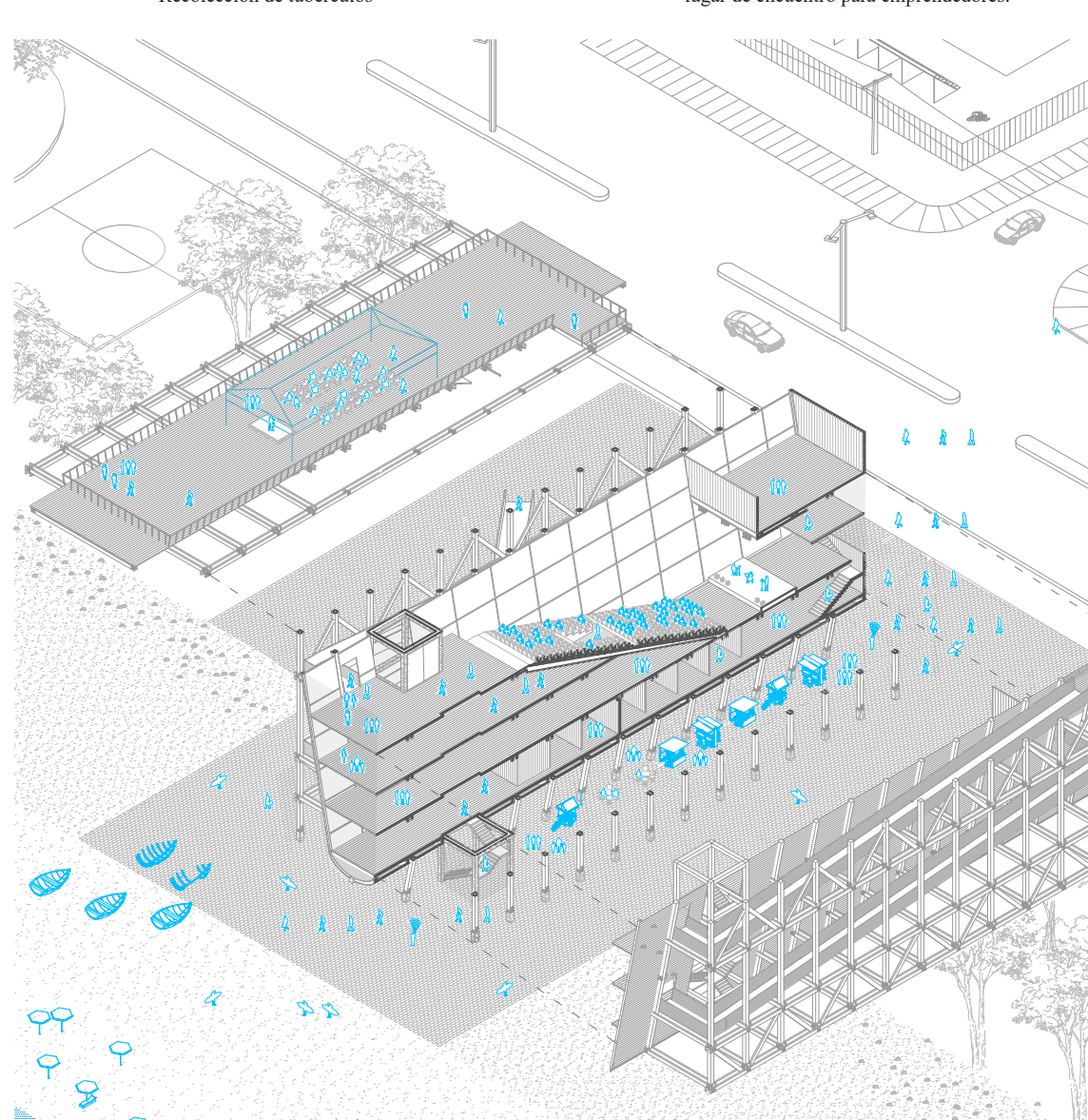
COSECHA Recolección de tubérculos
