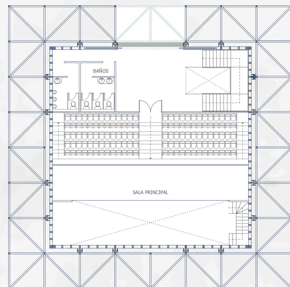
PLANTA NIVEL 2 ESC 1/200
