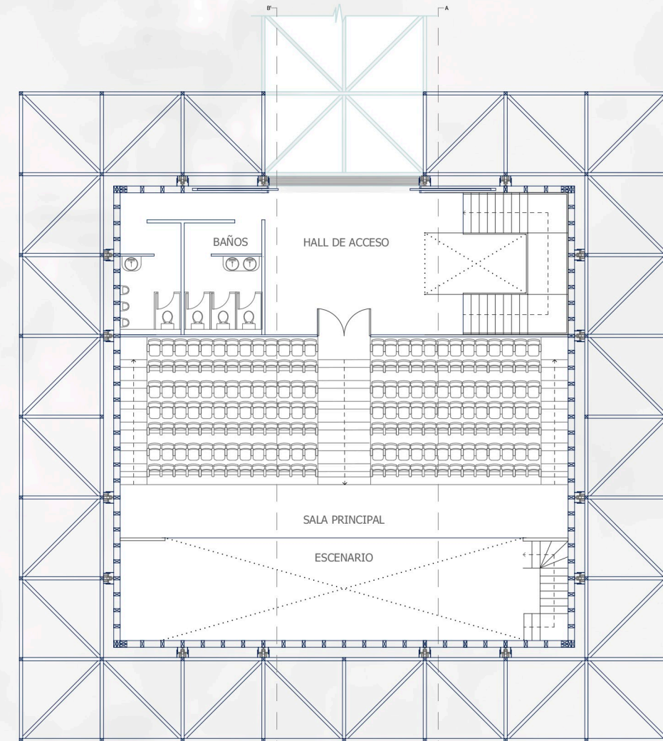
PLANTA NIVEL 2 ESC 1/200
