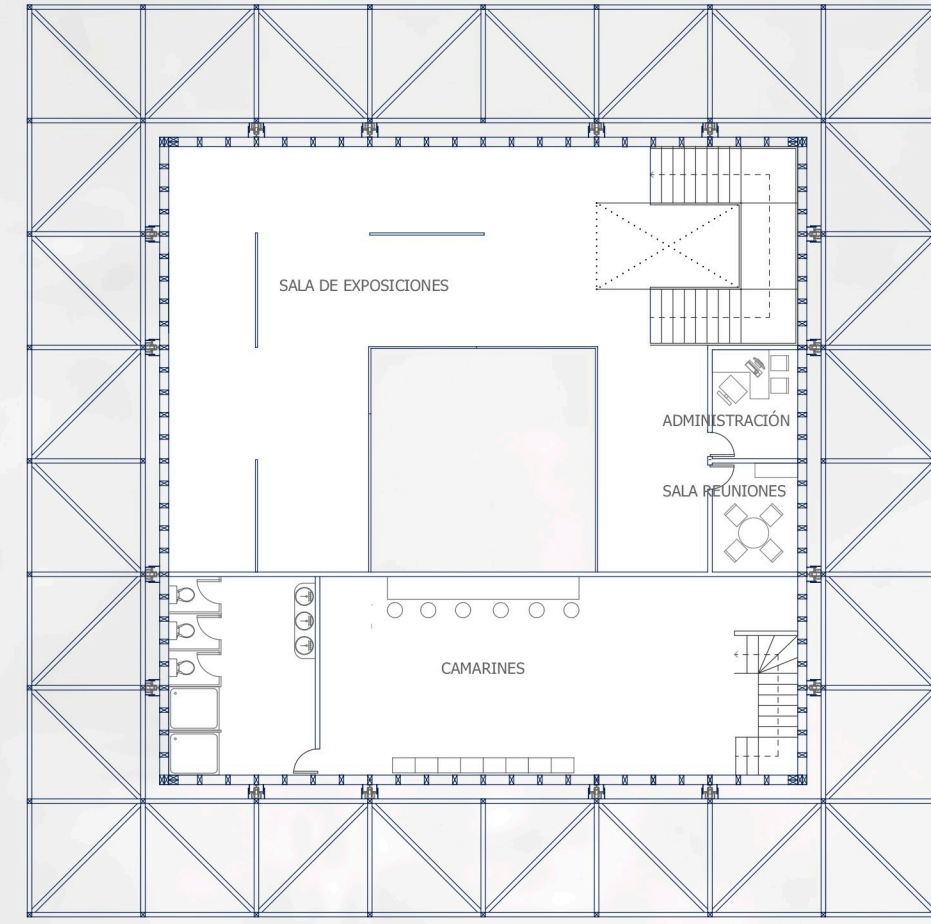
PLANTA NIVEL 1 ESC 1/200
