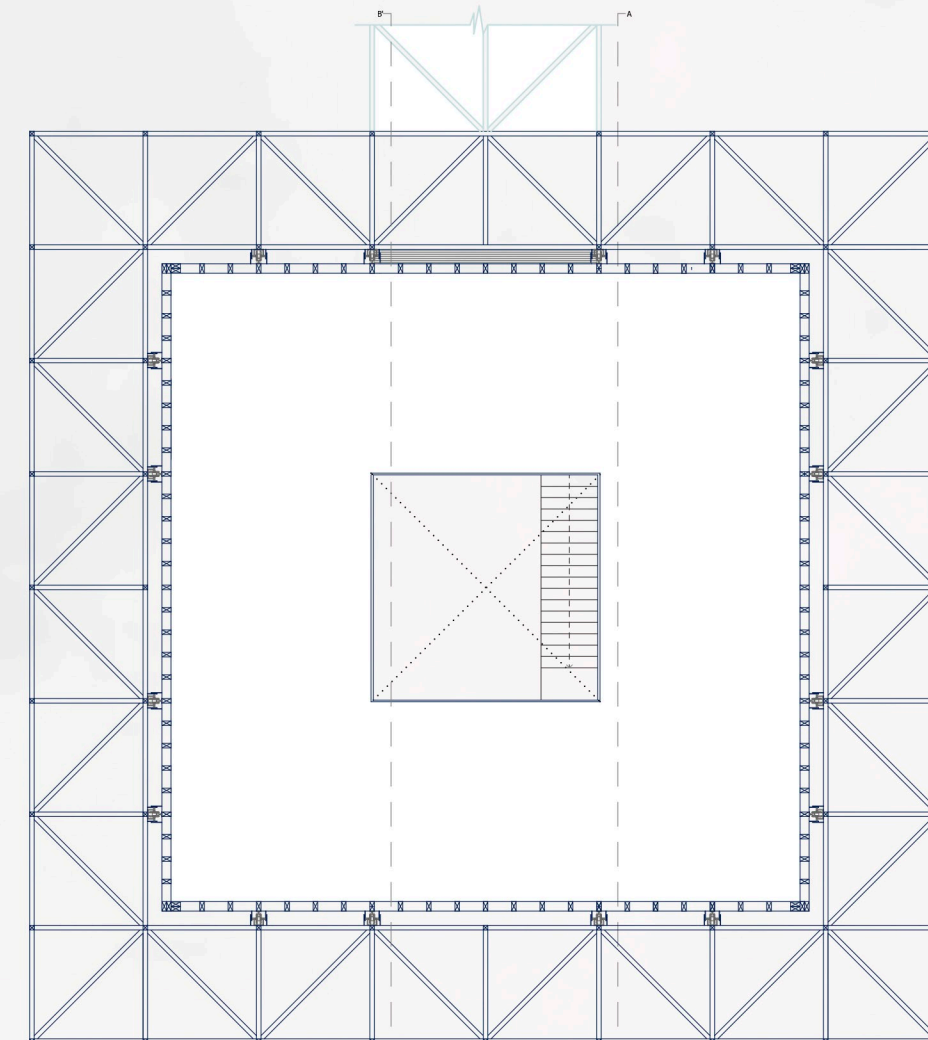
CUBIERTA ESC 1/500
