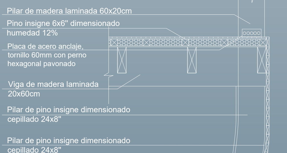
Detalle 4 Esc 1:50
