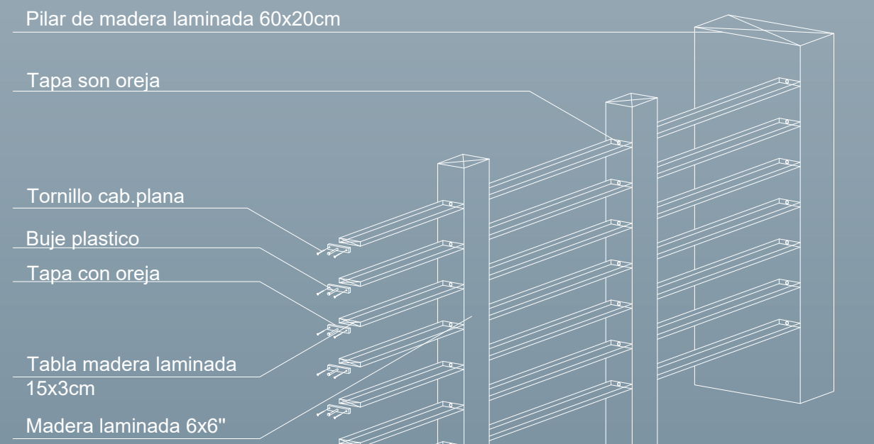
Detalle 2 Esc 1:30
