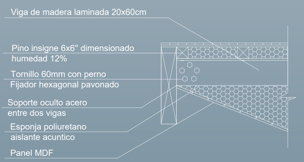
Detalle 3 Esc 1:30
