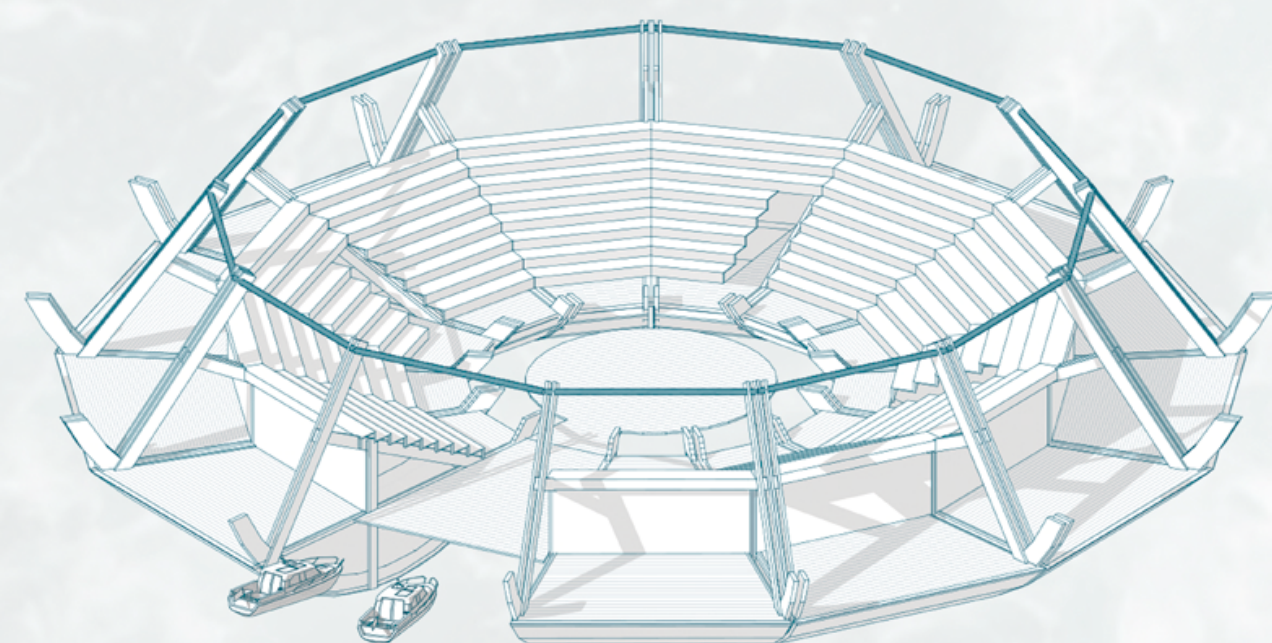
ESTRUCTURA TOTAL SIN MALLA
