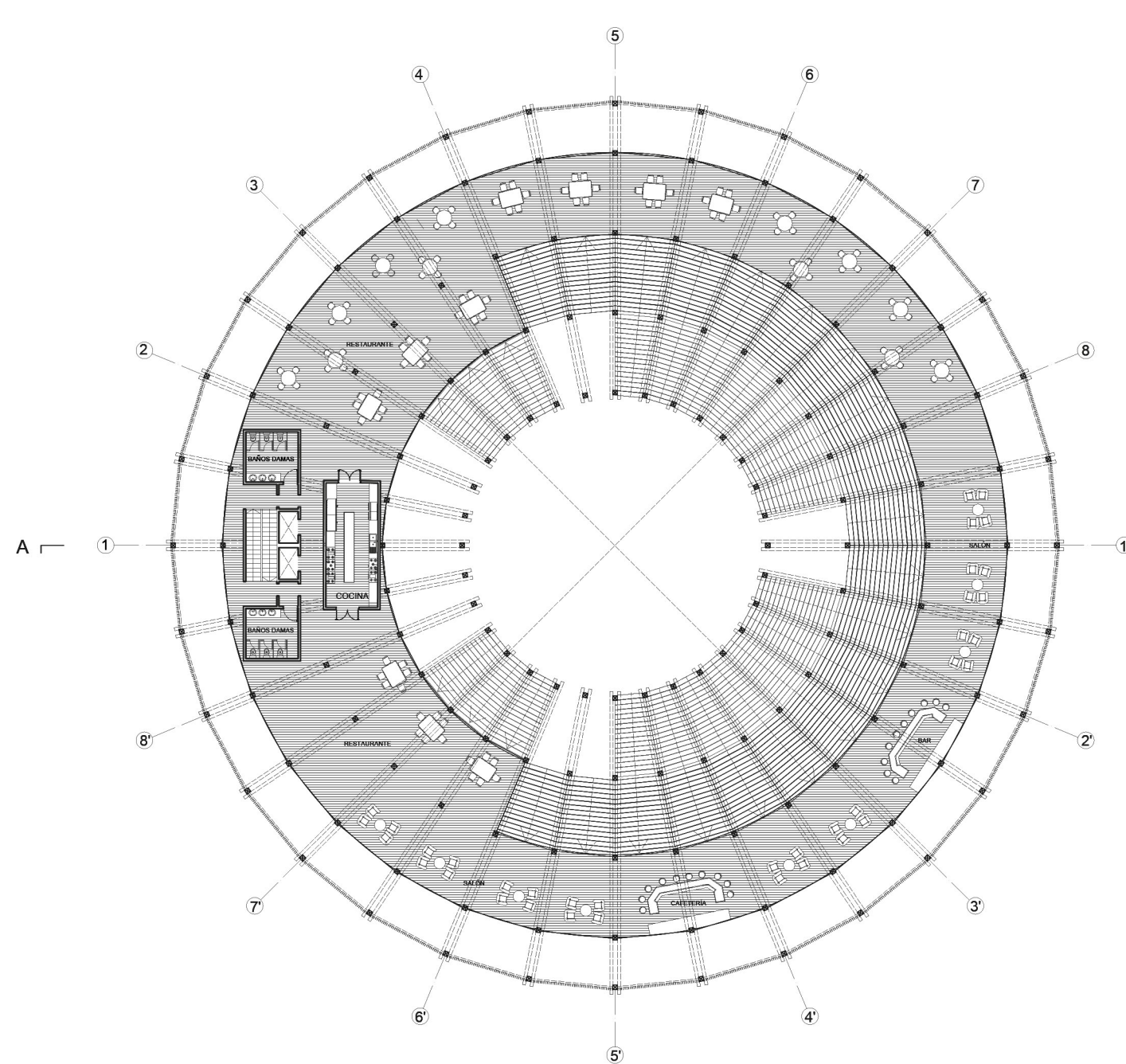
PLANTA NIVEL 02 RESTORANTE
