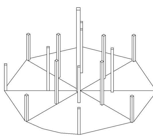
ESTRUCTURA DE CIRCO
