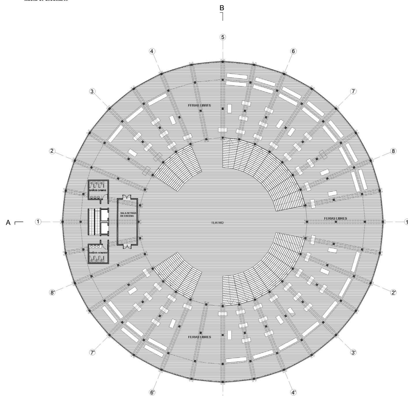
PLANTA NIVEL 01 FERIA
