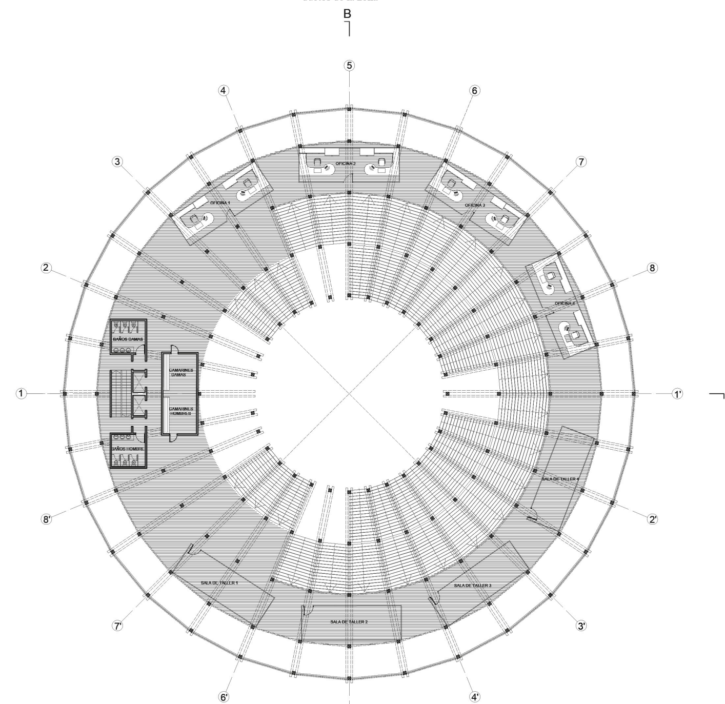
PLANTA NIVEL 03 OFICINAS - TALLERES
