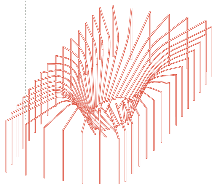
5. ESTRUCTURA PRINCIPAL DE MADERA LAMINADA CIMAS DEL PLIEGUE
