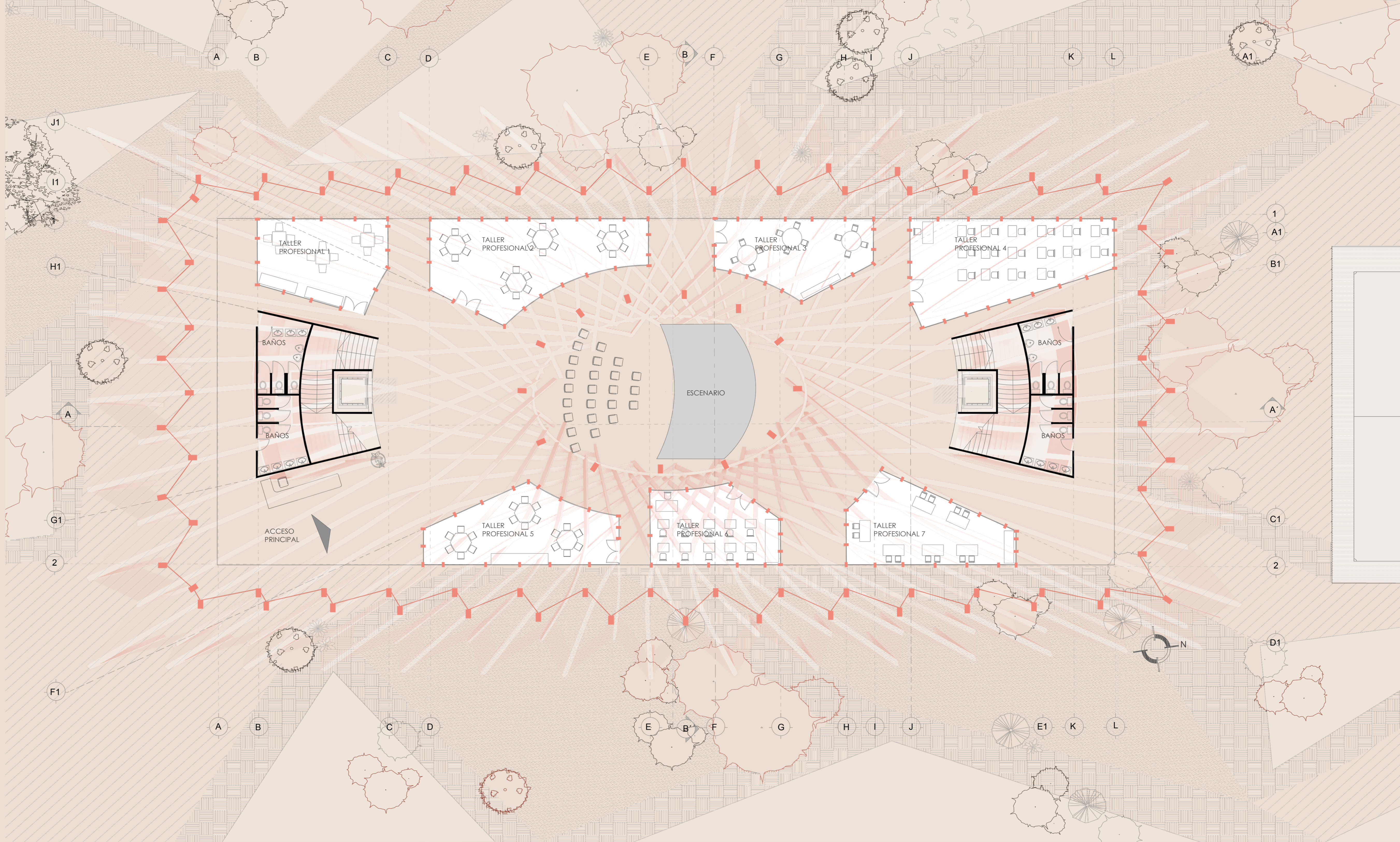
PLANTA DE ARQUITECTURA PRIMER NIVEL ESCALA 1 : 125
