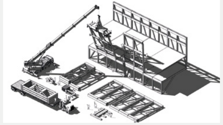
[4] Montaje de módulos y fachada
