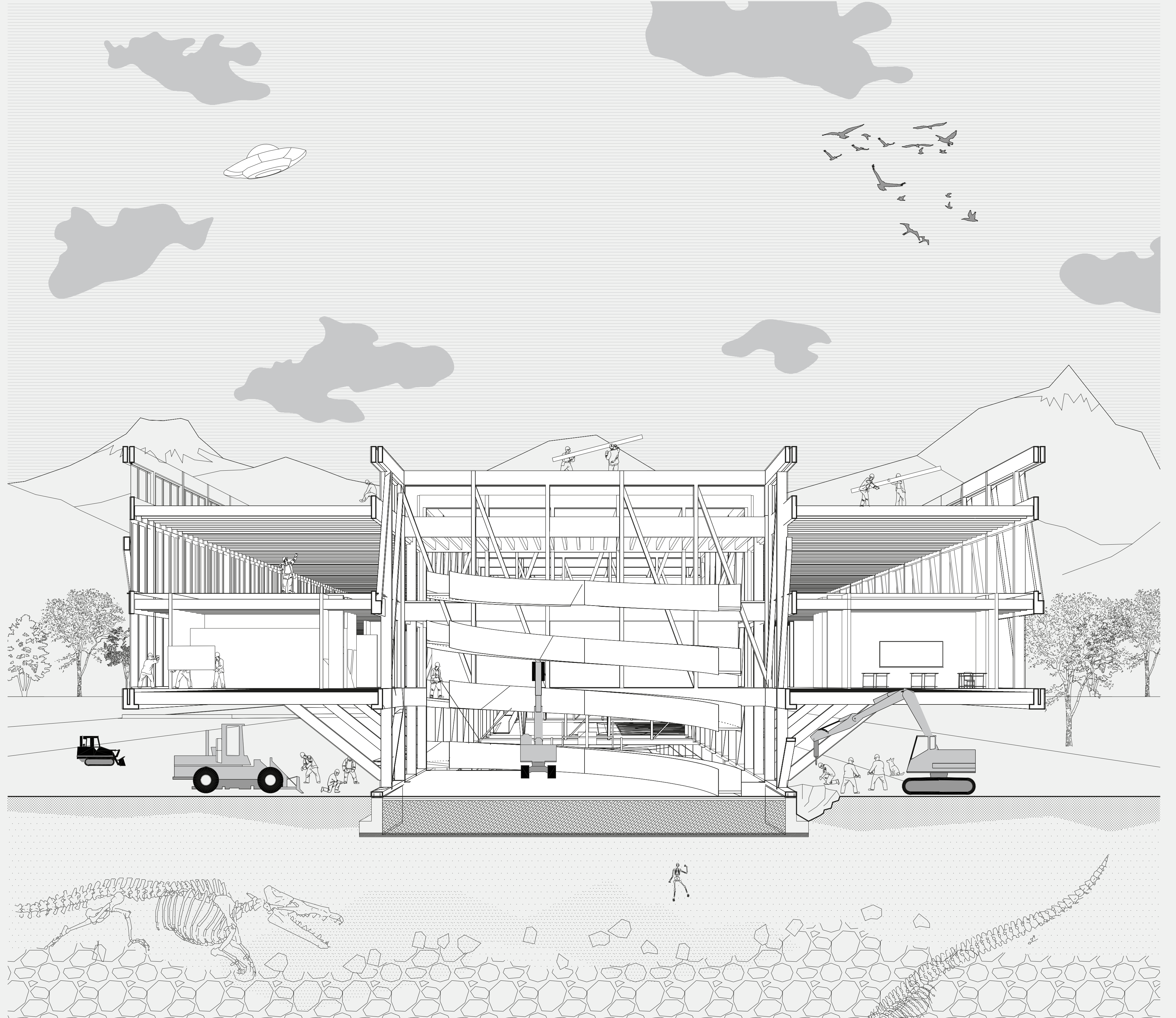
CORTE PERSPECTIVADO TRANSVERSAL | Patio Norte
