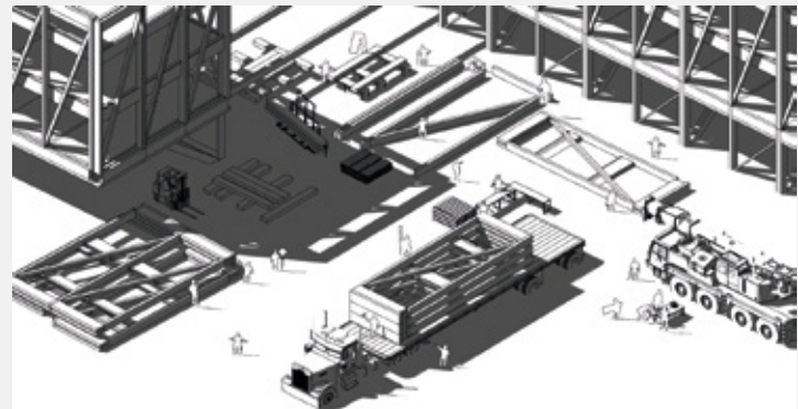
[2] Modelos prefabricados se cargan y salen del taller
