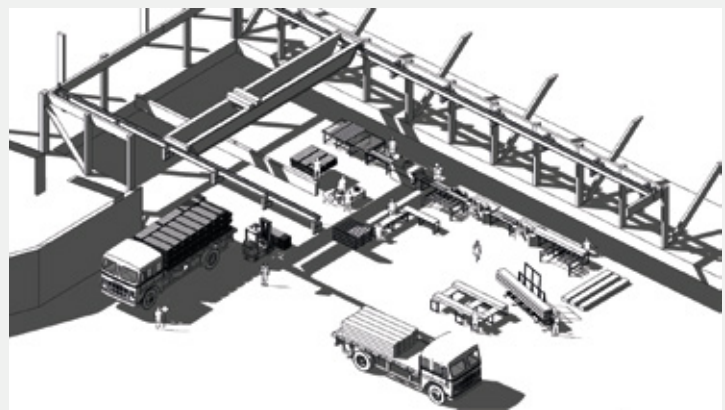
[1] Llegada de materia prima al taller
