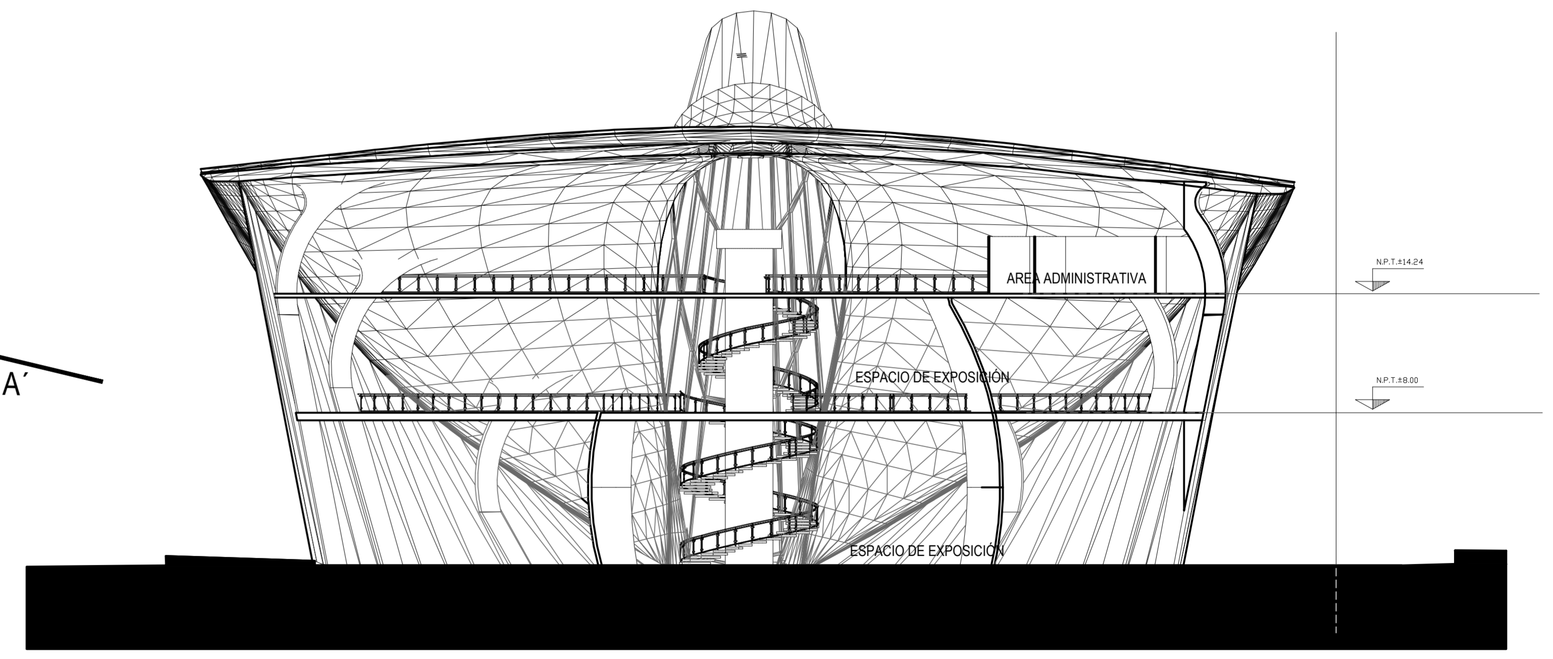
CORTE B - B' Esc 1: 200
