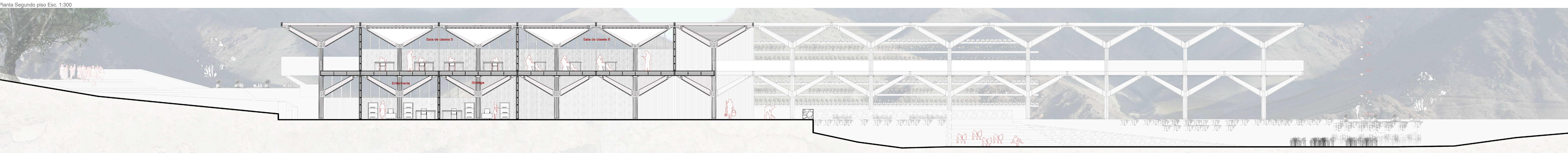
Corte de Proyecto B-B' Esc. 1:100
