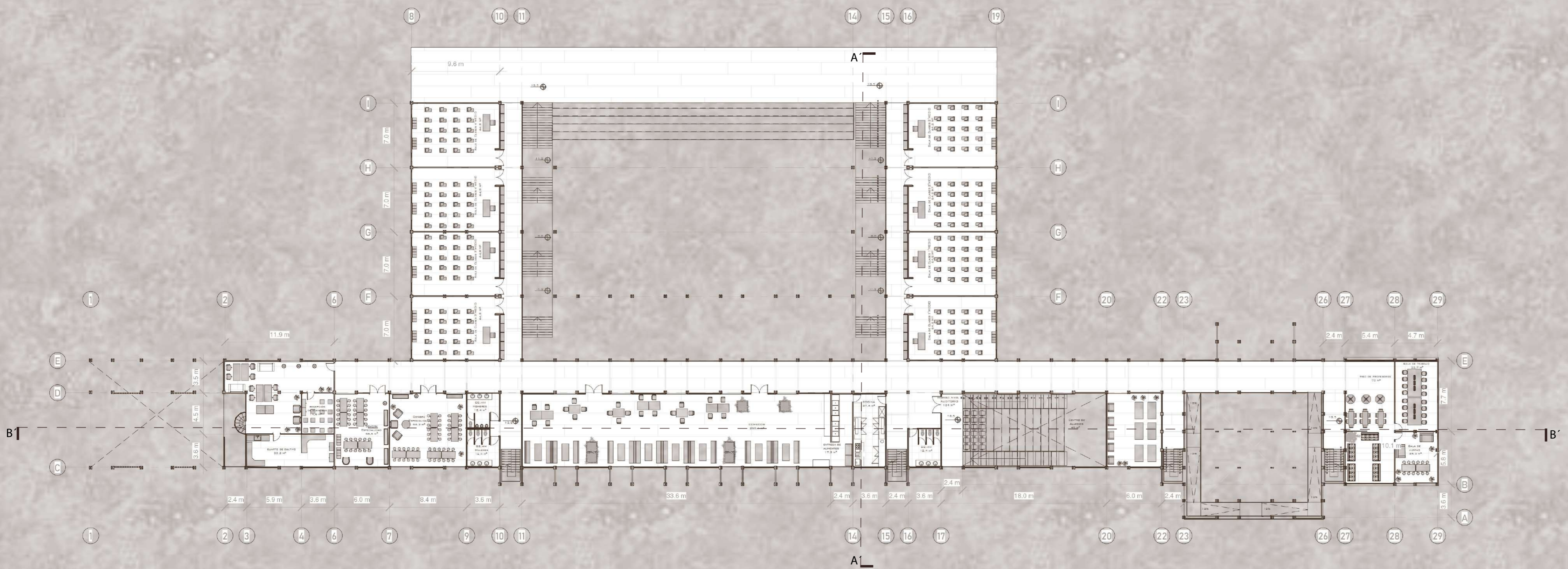
PLANTA NIVEL 2 / Esc 1:250
