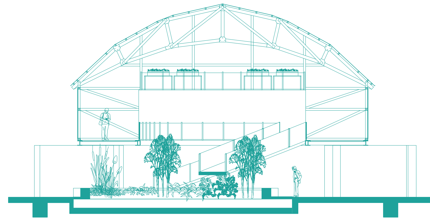
CORTE C ESC:1:125
