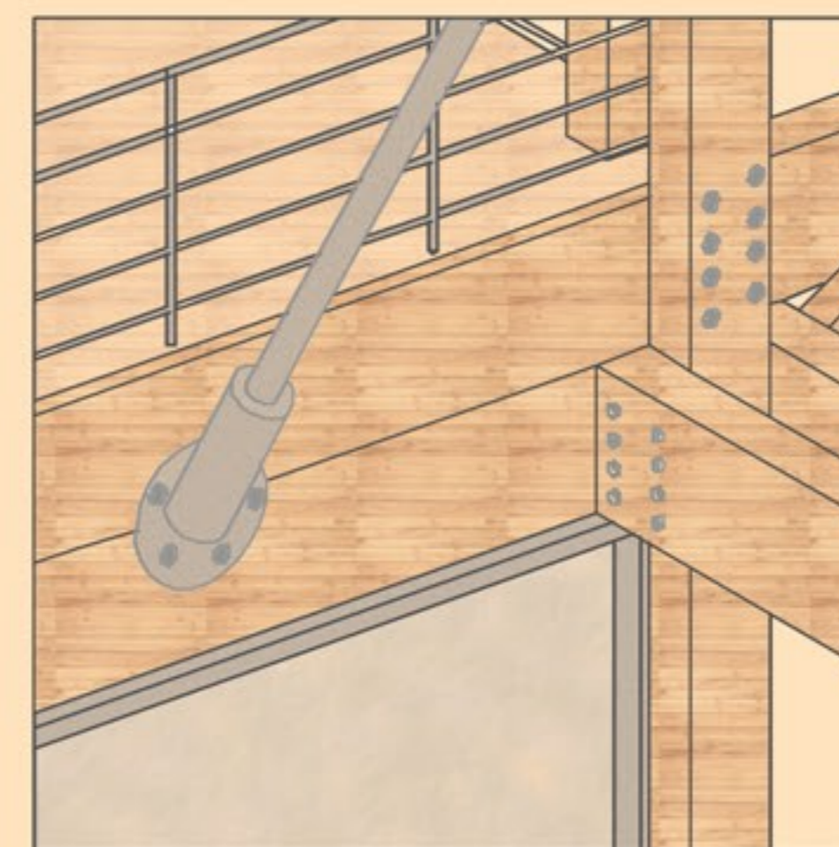
D1 - Encuentro Arriostamiento de cubierta O - 80x5mm Unión poste-viga Pernos O - 2 1/2 x 36"
