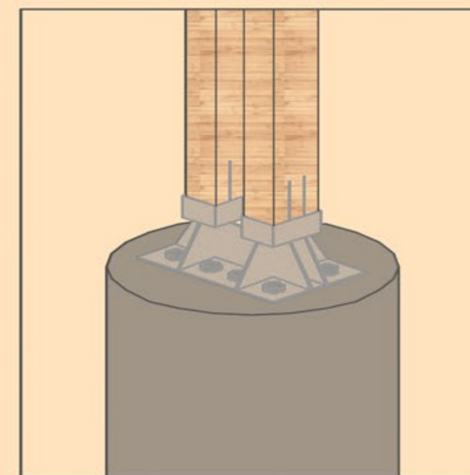
D3 - Encuentro Cimiento de acero sólido O - 1,2m x 10m Anclaje de acero inoxidable 5mm Pernos de anclaje O - 2 1/2 x 12"
