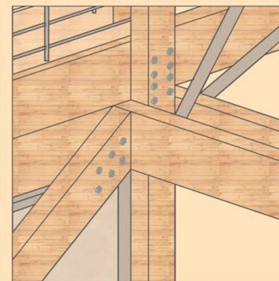
D2 - Encuentro Arriostamiento lateral y Unión poste-viga Pernos O - 2 1/2 x 36"
