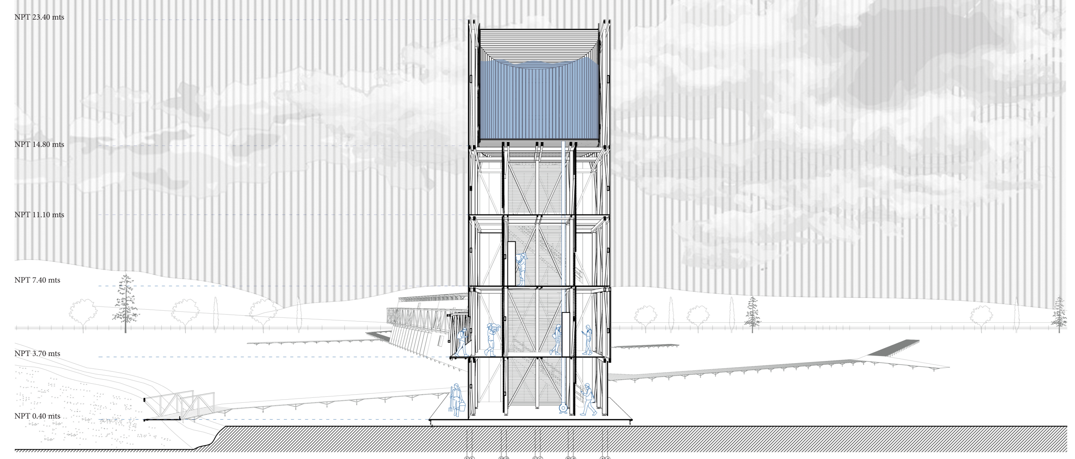
Corte torre de agua escala 1/125
