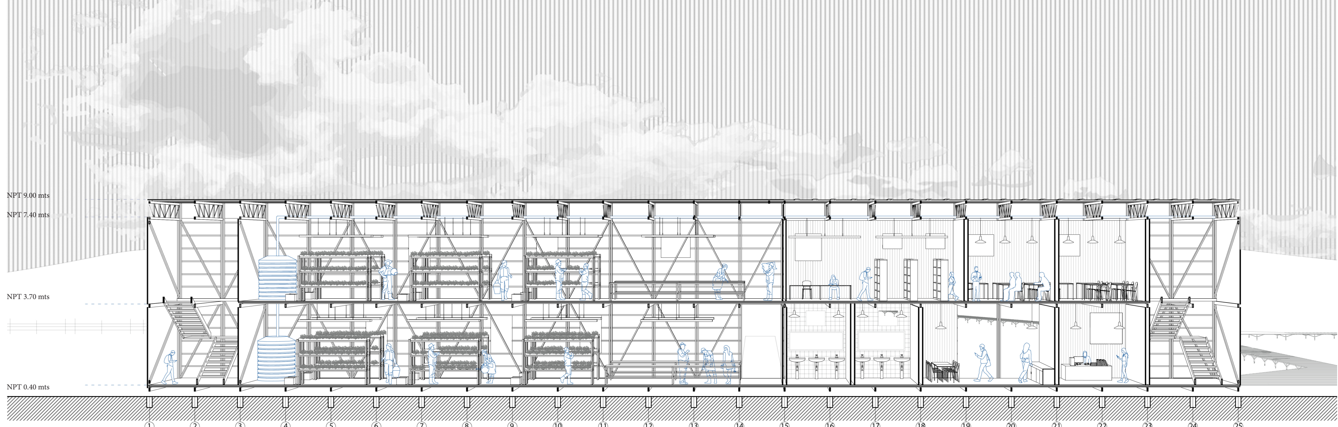
Corte edificio educacional escala 1/100
