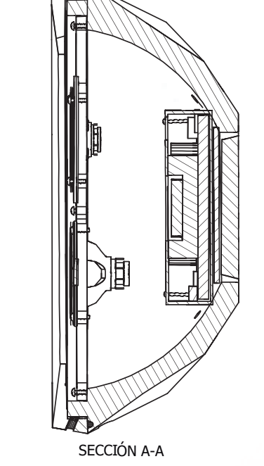
Corte "A"
