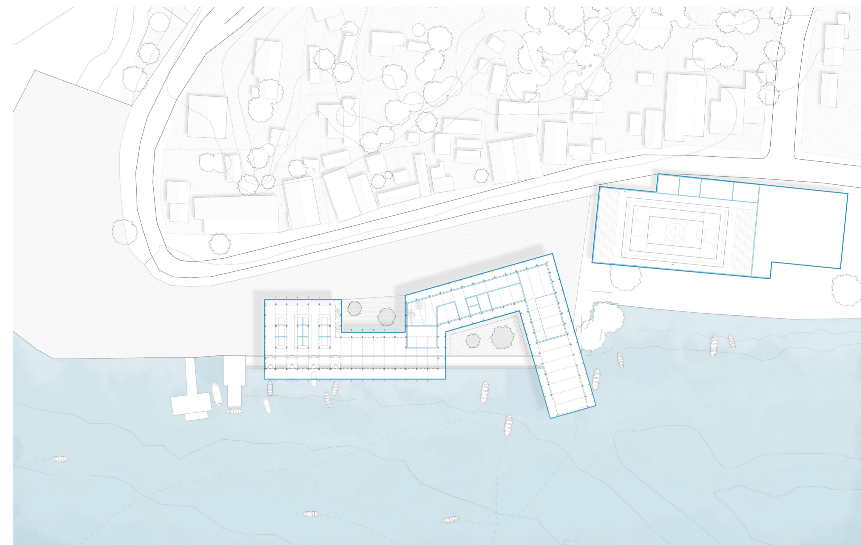
Emplazamiento ESC 1:750
