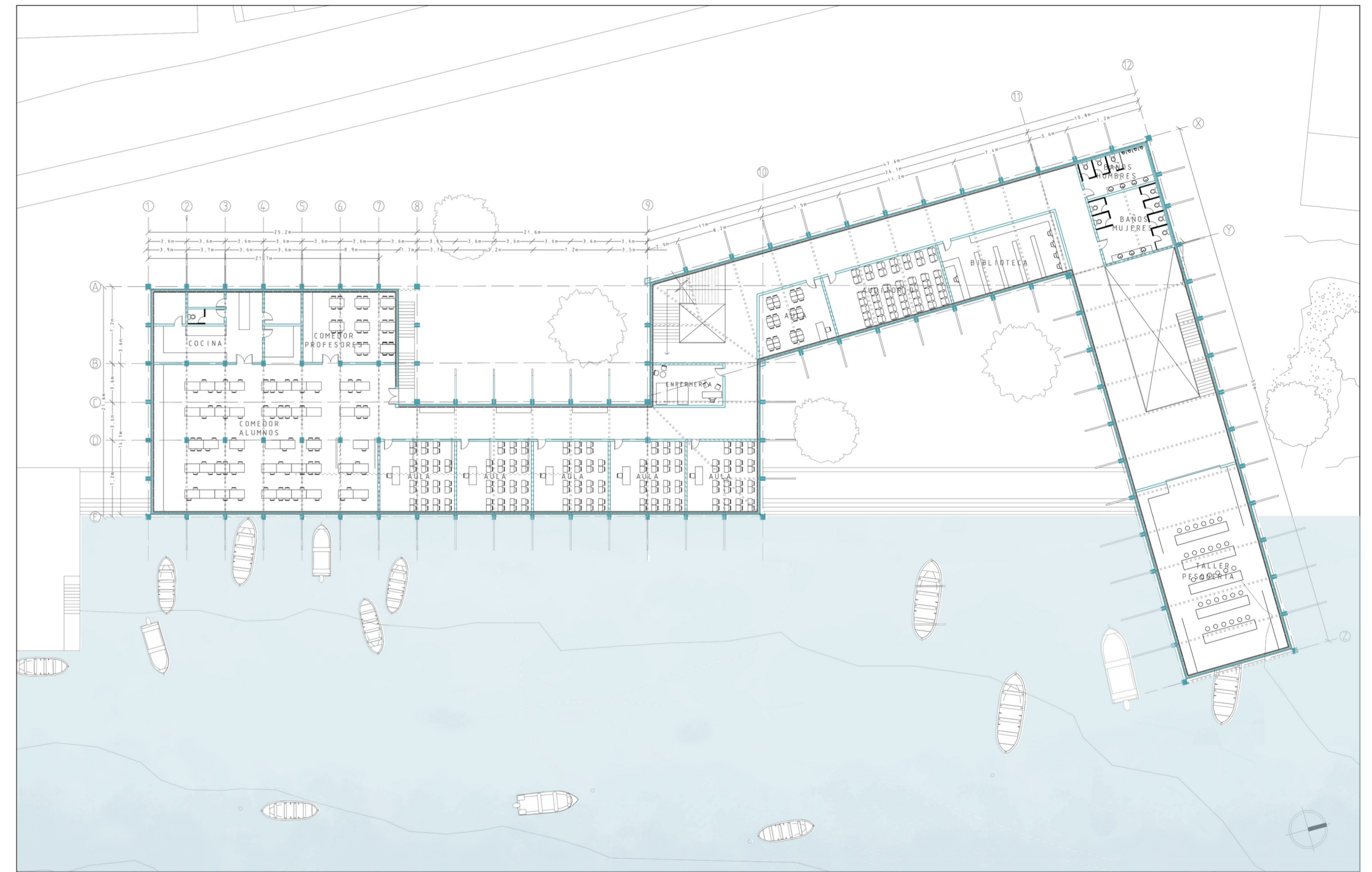
Segunda Planta ESC 1:300
