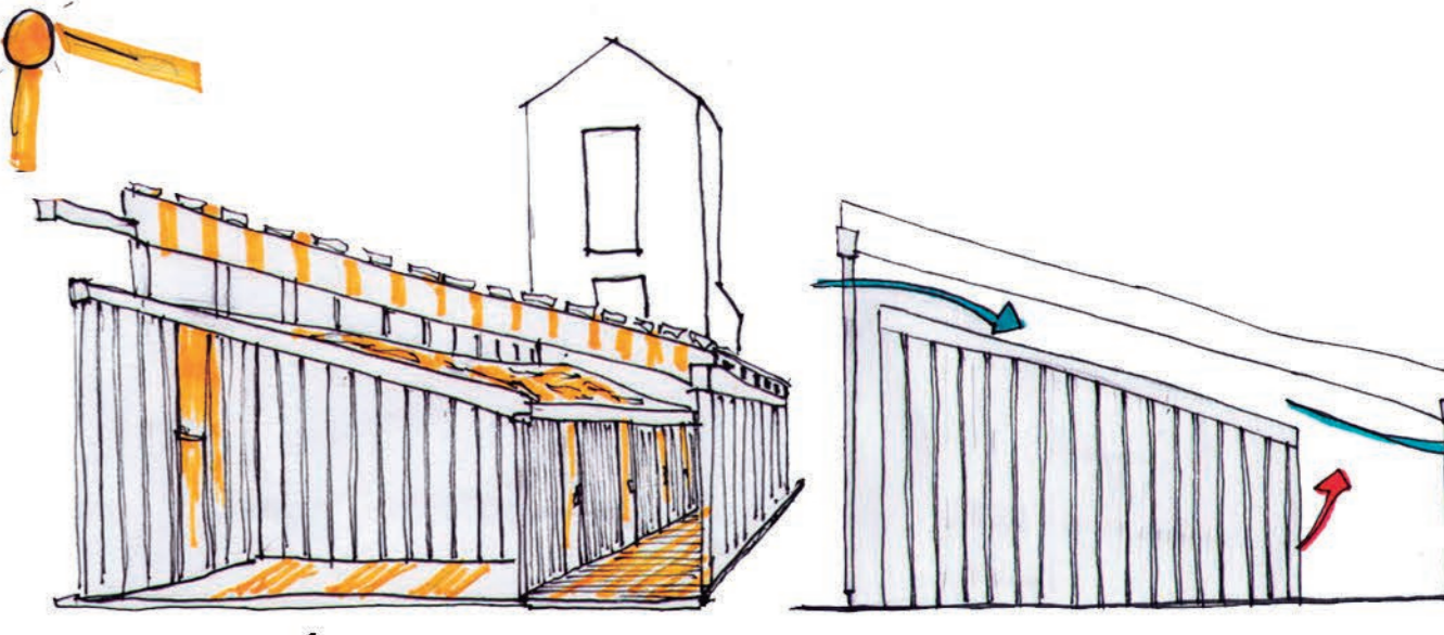
BALDOSA CLIMÁTICA PERIMETRAL A LA RUINA PARA EVITAR INUNDACIÓN
